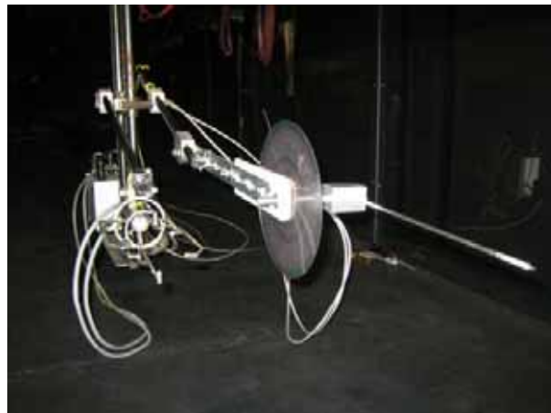
Photo.5 測定部
