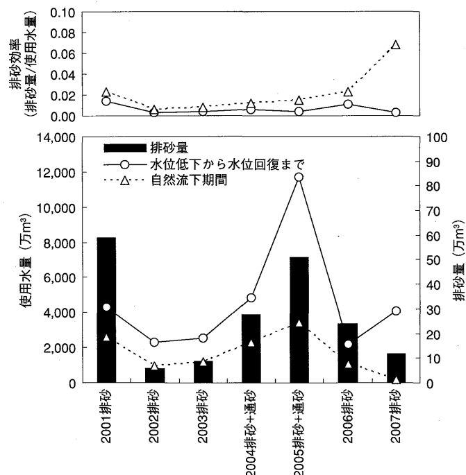
図―2 出し平ダムの2001～2007年の排砂・通砂時の排砂量・使用水量・排砂効率
