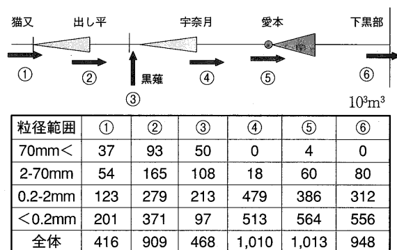
図-4 黒部川下流域における粒径別土砂収支（2006年7月）
