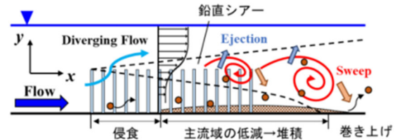
植生帯と土砂堆積の現象モデル
