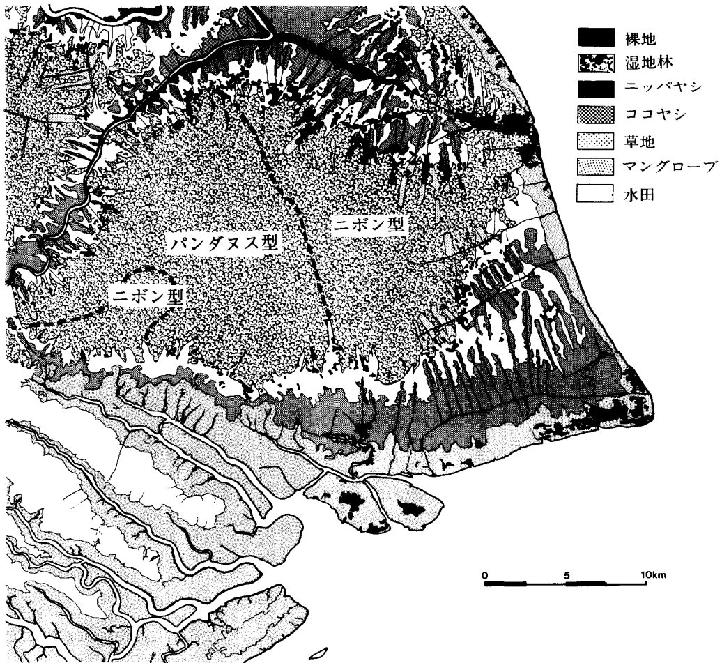
図3 1989年時の泥炭湿地林開発の様子 (TM画像より)
