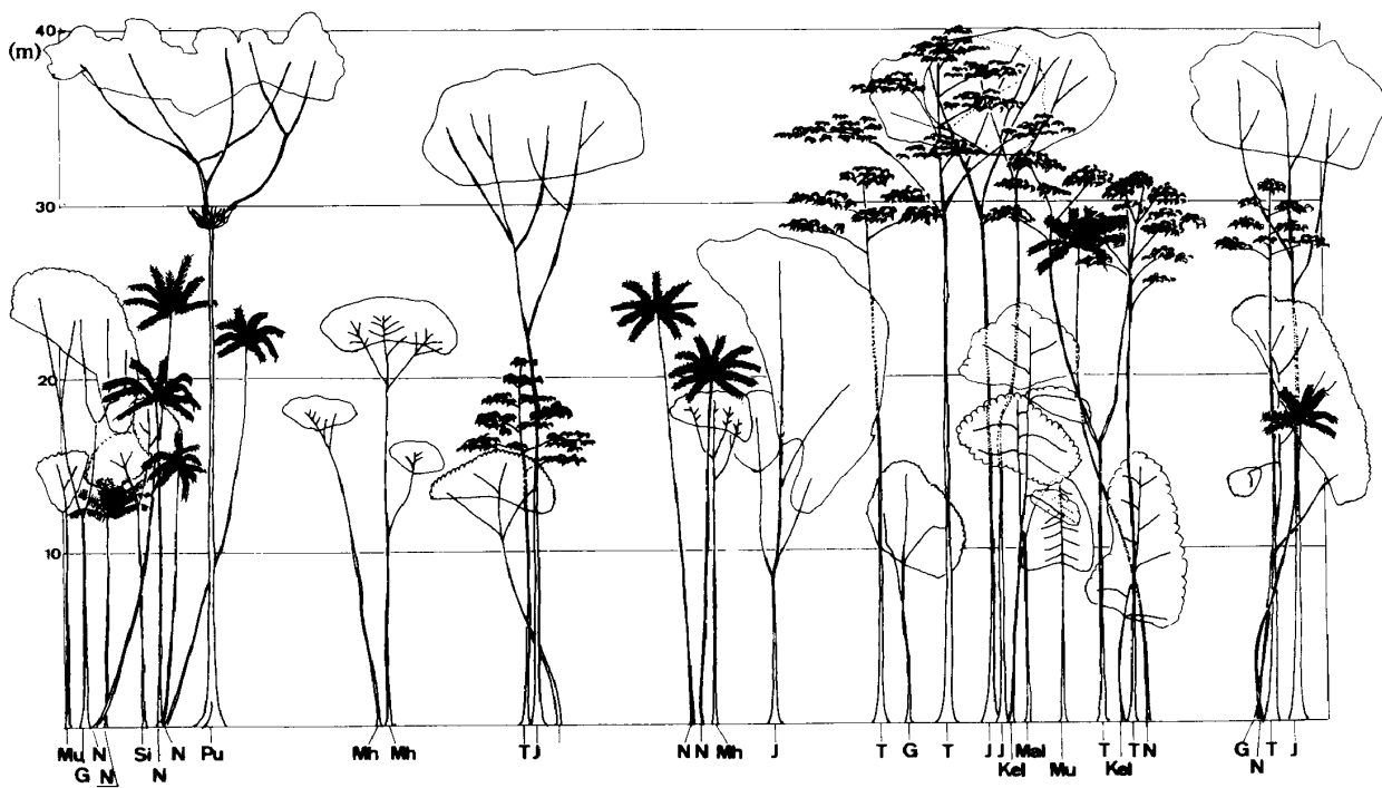
図 2-a 泥炭湿地林の相観図—ニボン型
