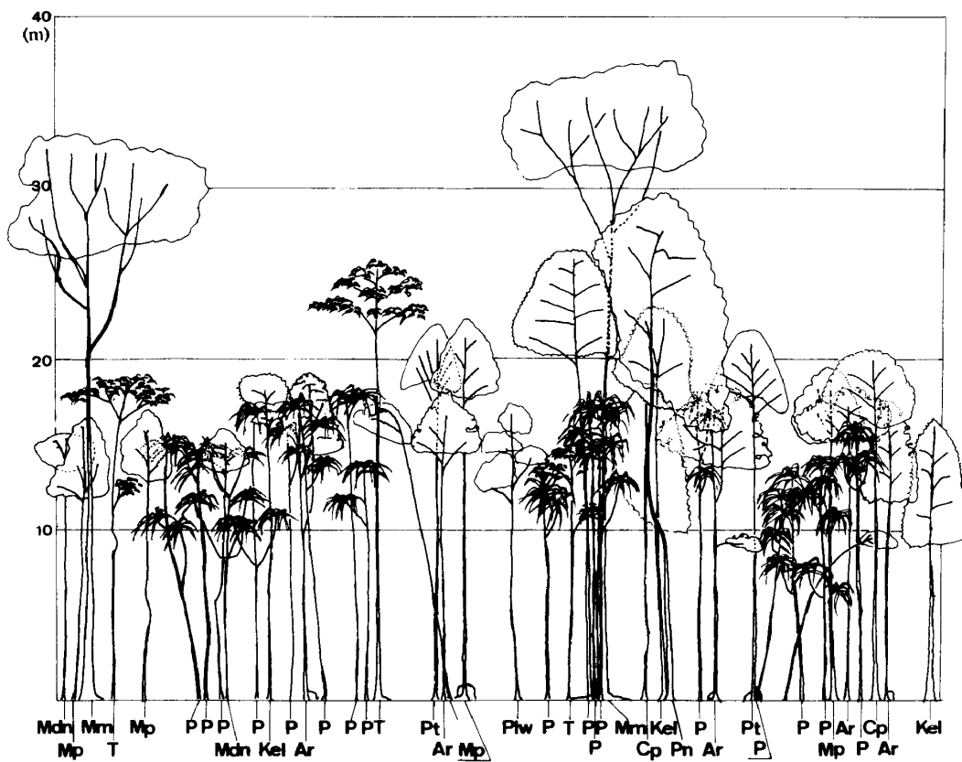
図 2-b 泥炭地湿地林の相観図—パンダヌス型
