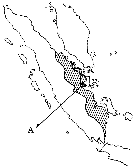
図1 調査地 Aの枠内が図3に示された範囲に相当。 斜線部は泥炭湿地帯。
