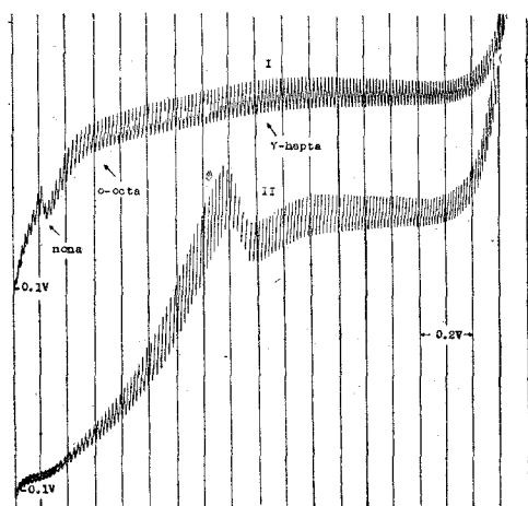
Fig. 11 : Polarogram(4).
