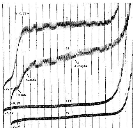
Fig. 8 : Polarogram(I).
