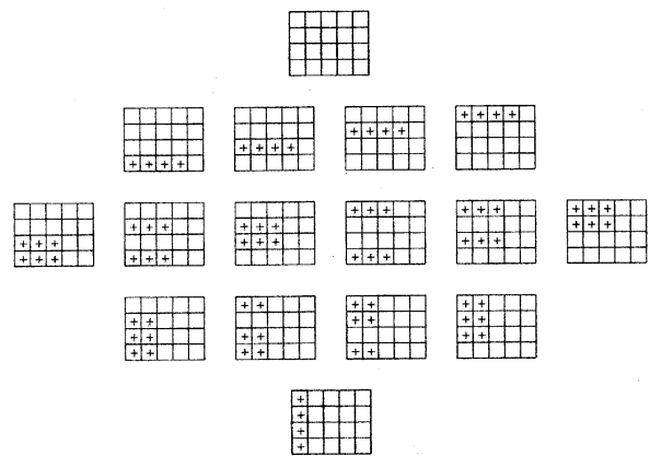
図 6: 証明に現れる主項
