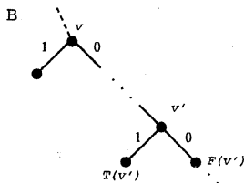
図4: 補題2の例
