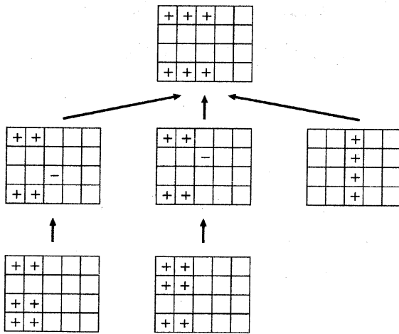
図 7: 主項の作り方
