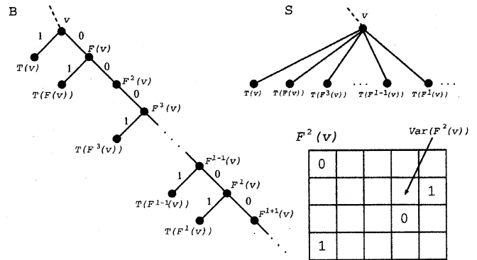
図 2: B から作られた S の一部分
