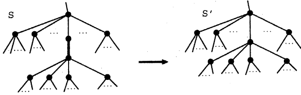
図 5: S の単純枝の除去
