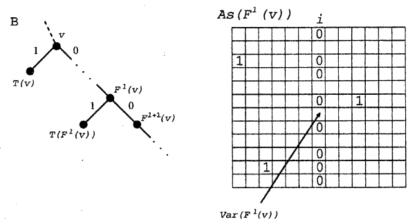
図 3: 頂点を CH(v) に加えるのをやめる条件
