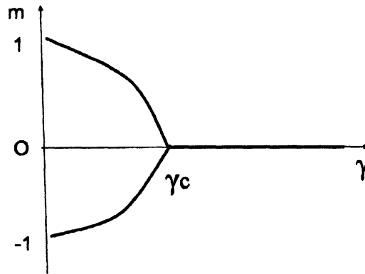
Figure 2: Order parameter and parameter \gamma (Ising model).
