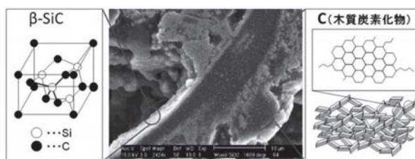
図4-33：木質バイオマス炭とSiCの複合体
