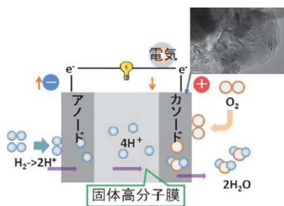
木材から燃料電池材料を作る仕組み
