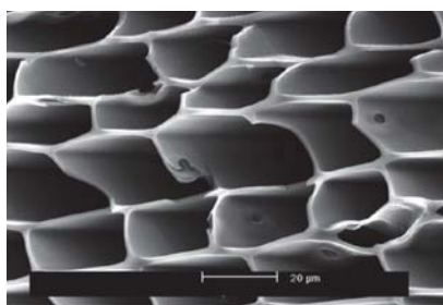
図 4-28：スギ木質炭素化物の細胞構造（畑，2007）
