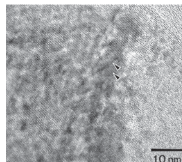
図 4-30：木炭中のミクロ黒鉛構造（2500℃）
