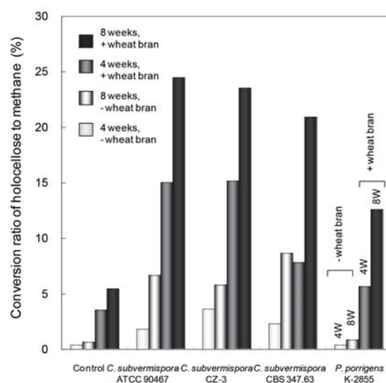
図 3-12: 白色腐朽菌処理スギチップのメタン発酵（坪田、渡辺, 2009; Amirta et al. , 2006）
