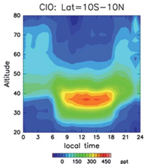
図2-18：赤道付近で見たClOの日変化を示す時間・高度断面図
