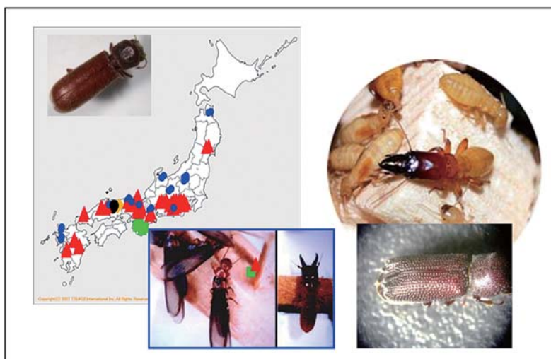
図6-10:新たな木材害虫達。左上:アフリカヒラタキクイムシとその分布域（赤のポイント（古川ら、2005より）、中央下:アメリカカンザイシロアリ、右上:ネバダオオシロアリ、右下:ホソナガシנקイ
