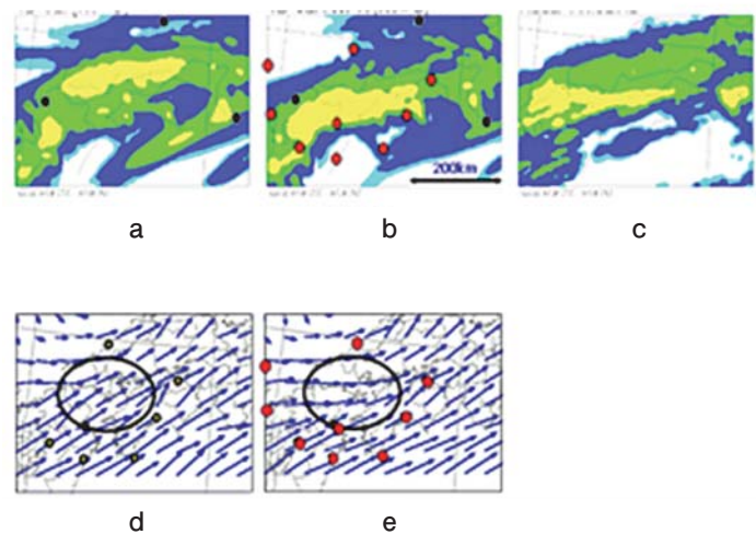
図 2-9：メソ数値予報モデル (MSM) による WINDAS インパクト (効果) 実験。(a) 2001 年 6 月 19 日 12UTC の初期値に WINDAS 観測値を使用せずに予報した 15UTC における 3 時間積算降水量。(b) 12UTC の 6 時間前から WINDAS 観測値をデータ同化して予報した 15UTC における 3 時間積算降水量。(c) 15UTC におけるレーダー・アメダス解析雨量の 3 時間積算降水量。(d) (e) それぞれ (a) (b) に対応する 850hPa における風の予報値
