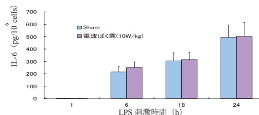
図3-20：U937細胞による IL-6 分泌量 (10W/kg 4時間ばく露)
