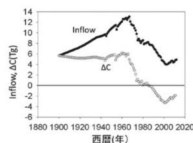
図 4-3：HWP 炭素貯蔵庫への流入量 Inflow と吸収量 \Delta C の関係（国産材のみの場合、HL=35 年）
