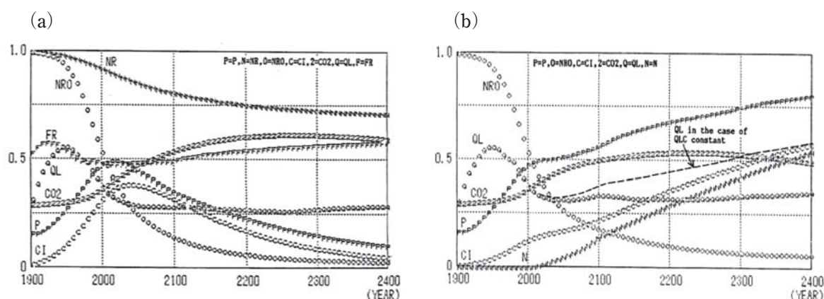
図 3-4：ローマクラブによる成長の限界シミュレーションに SPS を加味したシミュレーション結果 (Yamagiwa, 1992)
