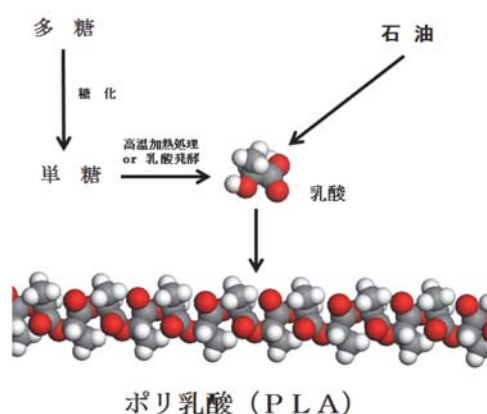
図 4-17：ポリ乳酸（PLA）の合成
