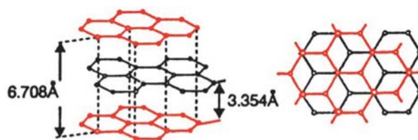
図 4-27：黒鉛の結晶構造
