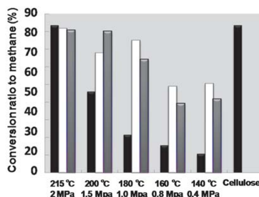
図 3-13: 白色腐朽菌・爆砕複合処理によるブナ材のメタン発酵（坪田・渡辺, 2009）
