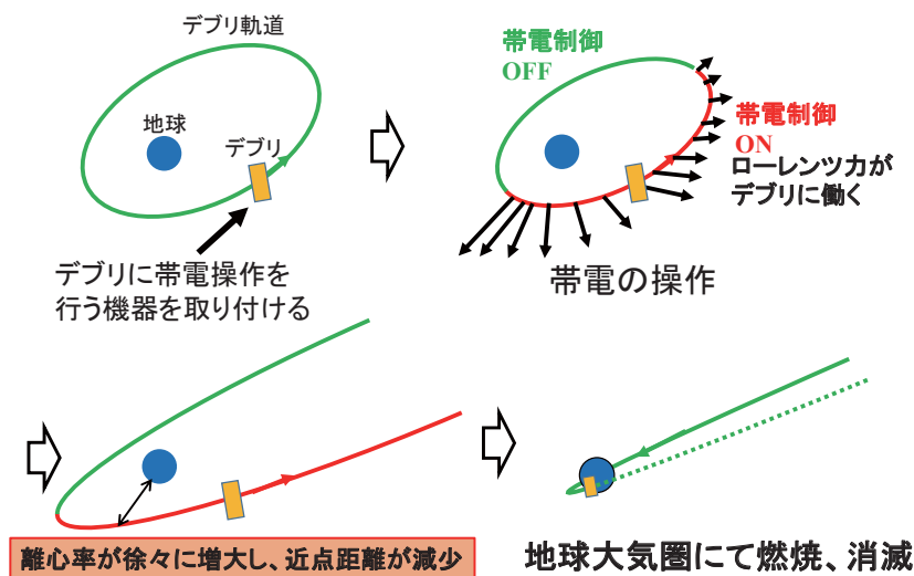
図 5-24：帯電制御によるデブリ除去
