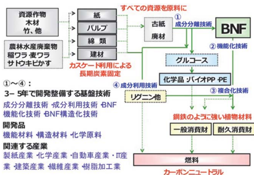
図 4-25：地域自立型バイオマスコンビナートを目指して（JCII・BNF 勉強会資料を改変）
