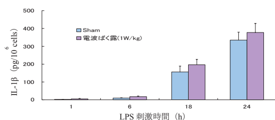
図3-17：U937 細胞による IL-1 \beta 分泌量 (1W/kg 4時間ばく露)
