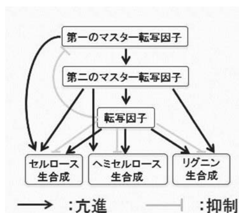
図 2-26：木質バイオマス形成の転写制御システムの概念図
