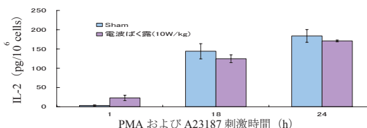
図3-22：Jurkat 細胞による IL-2 分泌量 (10W/kg 4時間ばく露)
