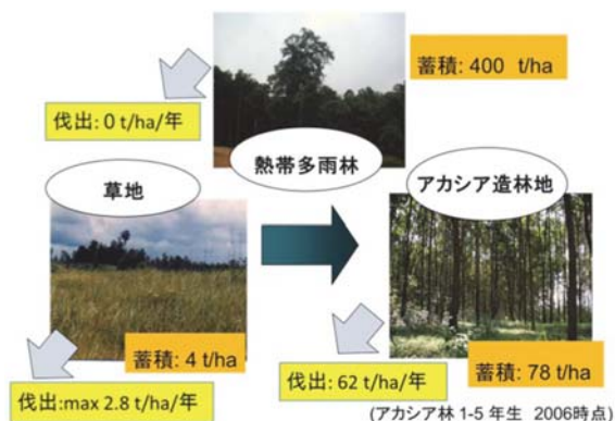
図 4-6: 天然林、人工林、草地のバイオマス蓄積量（ストック）と原木伐採（フロー）（川井 2012）
