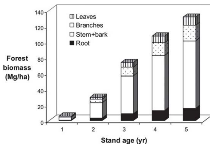
図 4-5：アカシヤマンギウム林木のバイオマス蓄積量と樹齢の関係
