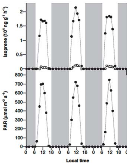
図 2-5: イソブレン放出の日周性 (Saito & Yokouchi, 2006)
