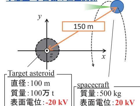
図 5-14：クーロンアトラクタによる小惑星ランデブー
