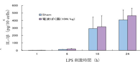
図3-18：U937 細胞による IL-1 \beta 分泌量 (10W/kg 4時間ばく露)
