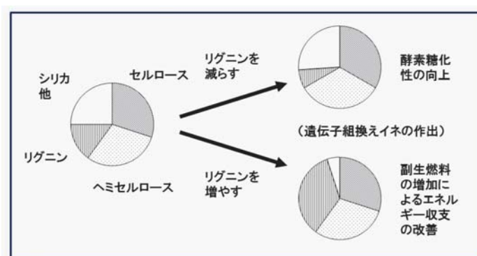
図 2-27: イネのリグニン量の制御の代謝工学 (イネ: 実用植物兼イネ科エネルギー植物のモデル)
