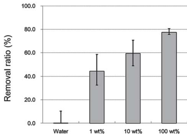
図 2-33：純水, JPAL® (1wt%), JPAL® (10wt%), JPAL® (100wt%) を洗浄剤とした場合の不織布の除染効果。
