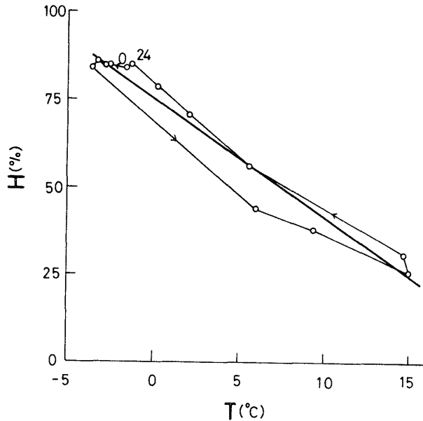
Fig. 20 湿度・温度の日変化(1974年1月26日) ビニルシート内装, 白丸: 2時間毎の 観測値, 太線: 回帰直線( H = -3.42T + 75.6 , r = -0.980 )
