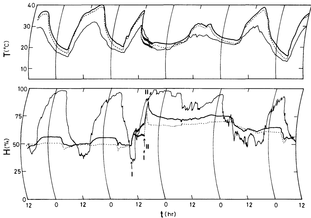
Fig. 10 住宅内気候の経時変化 (1974年6月15日～20日)
