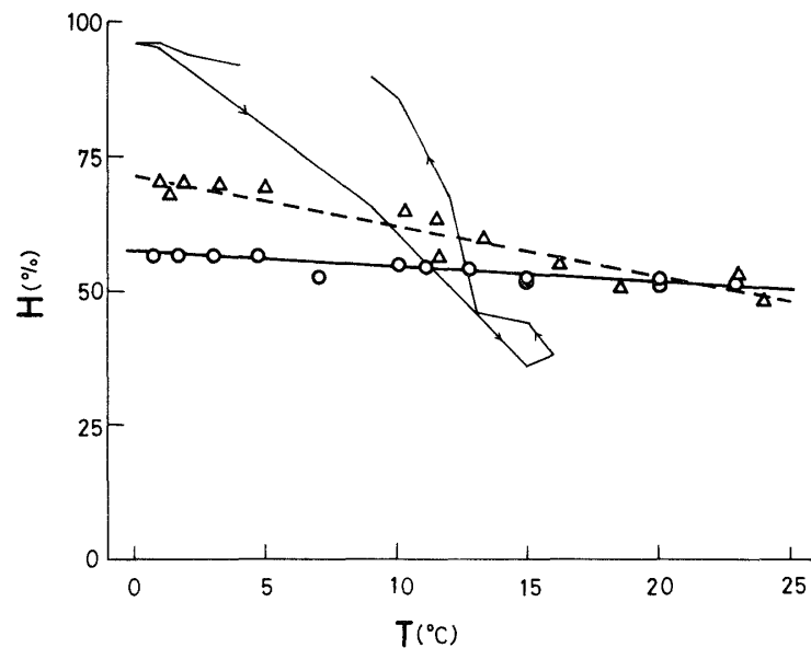
Fig. 22 湿度・温度の日変化 (1974年2月19日) 白丸: 合板内装, 三角: フェノール・メラミン樹脂板内装, 細線: 百葉箱
