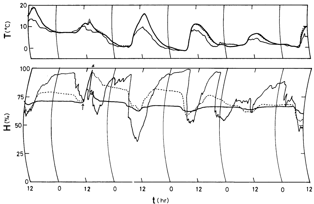
Fig. 16 住宅内気候の経時変化 (1975年12月8日～13日) 太線：合板内装，点線：メラミン美粧合板内装，細線：百葉箱
