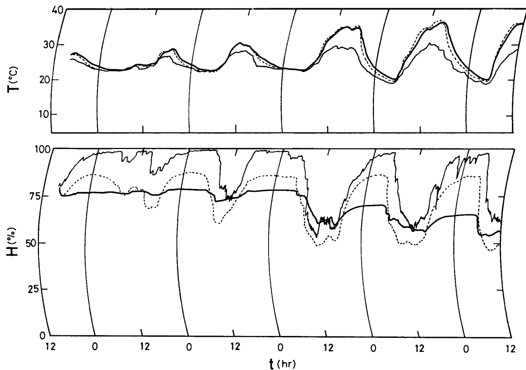
Fig. 12 住宅内気候の経時変化 (1974年7月17日～22日)
