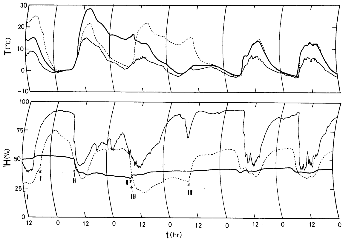
Fig. 15 住宅内気候の経時変化 (1975年2月24日～3月1日) 太線：合板内装，点線：メラミン美粧合板内装，細線：百葉箱
