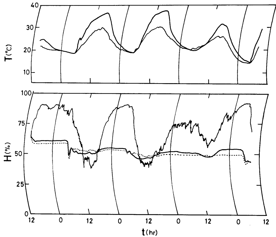
Fig. 11 住宅内気候の経時変化 (1974年6月11日～15日)
