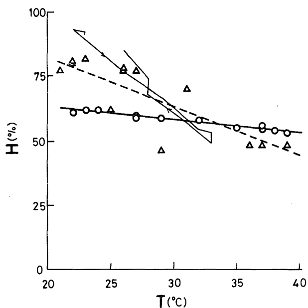
Fig. 25 湿度・温度の日変化(1974年8月6日) 白丸：合板内装，三角：メラミン美粧合板内装，細線：百葉箱
