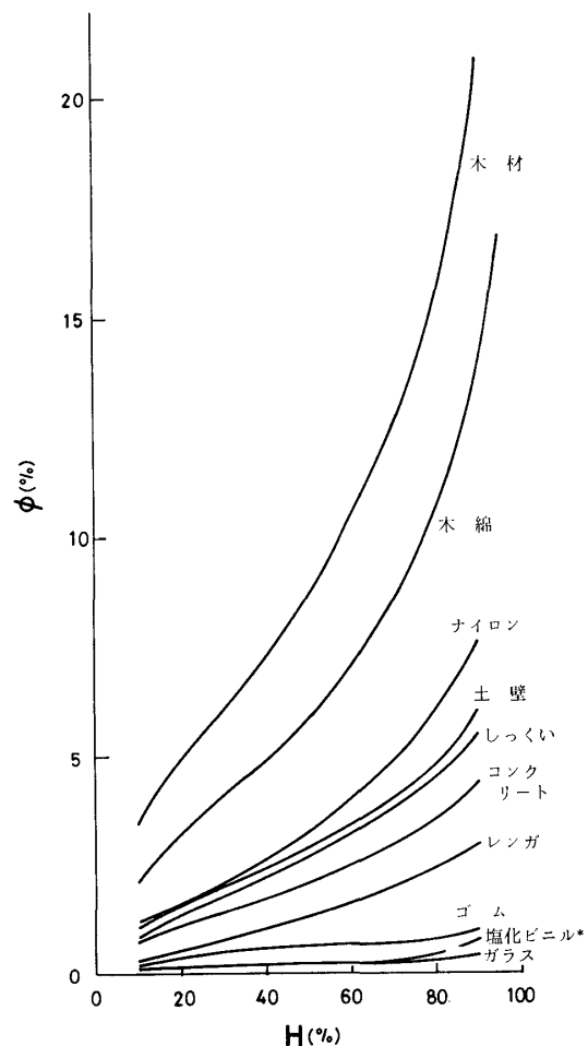
Fig. 3 材料の吸着等温線 (20°C) * 30°C
