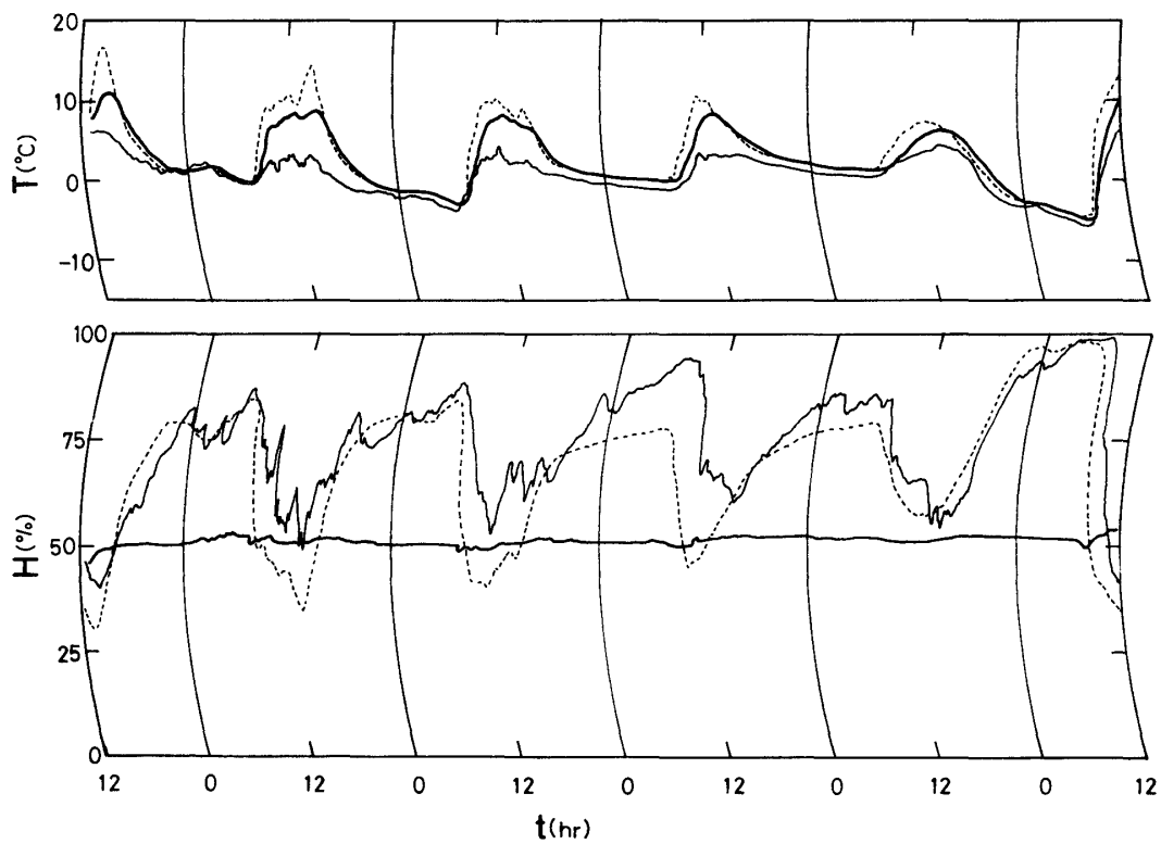
Fig. 8 住宅内気候の経時変化 (1974年1月27日～2月1日)
