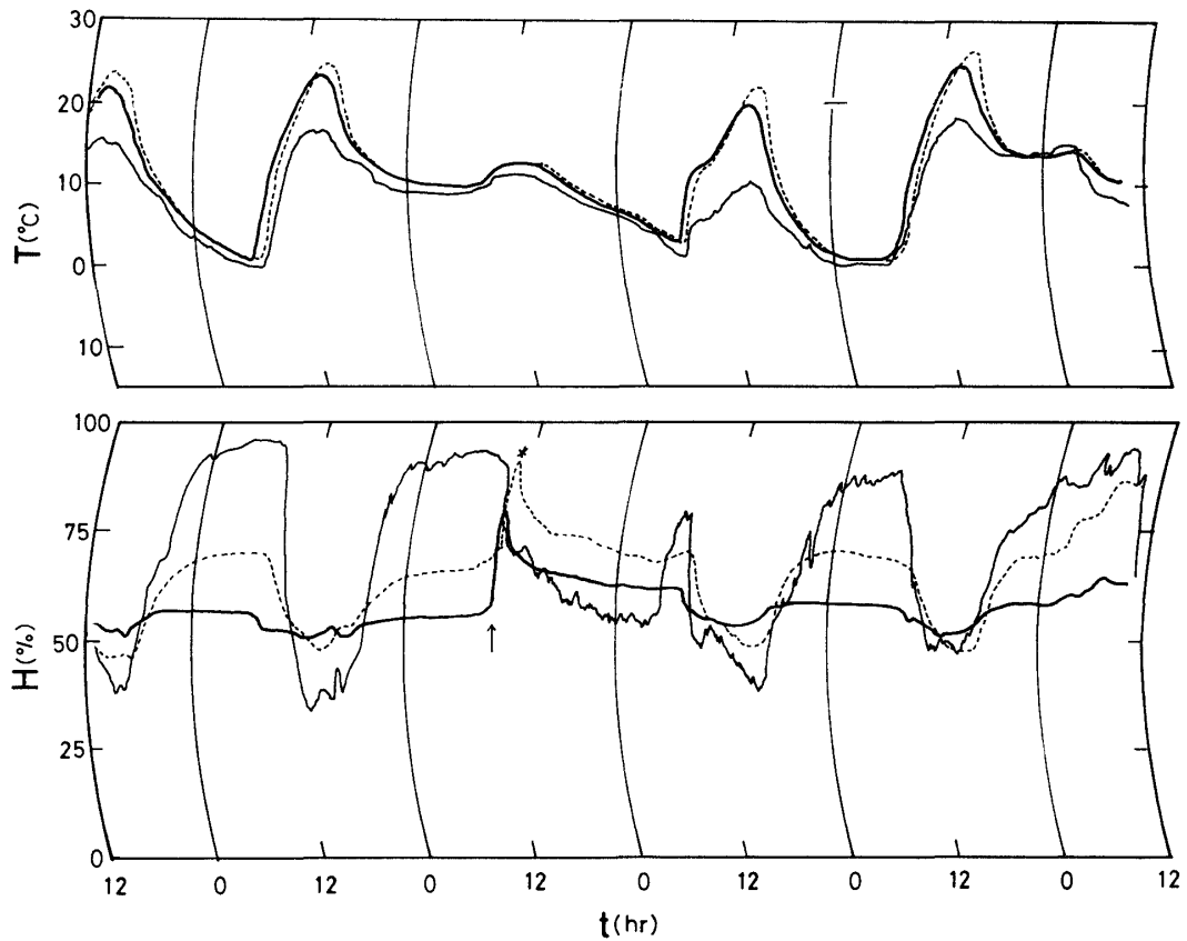
Fig. 9 住宅内気候の経時変化 (1974年2月18日～23日)
