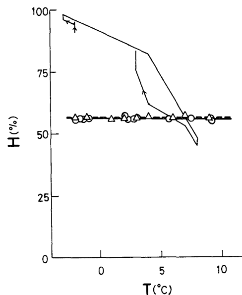
Fig. 24 湿度・温度の日変化(1973年12月31日) 白丸：合板内装，三角：珪酸カルシウム板内装，細線：百葉箱
