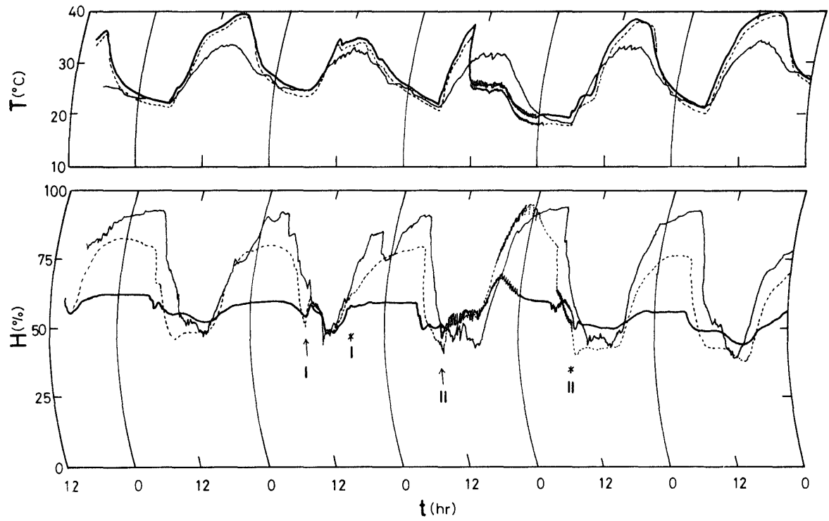
Fig. 13 住宅内気候の経時変化 (1974年8月5日～10日) 太線：合板内装，点線：メラミン美粧合板内装，細線：百葉箱
