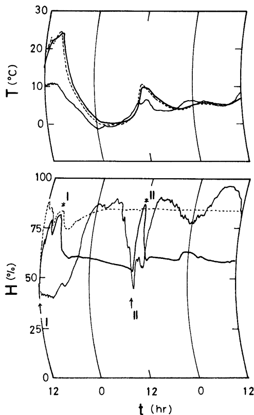
Fig. 17 住宅内気候の経時変化 (1975年3月4日~6日) 太線：合板内装，点線：メラミン美粧合板内装，細線：百葉箱
