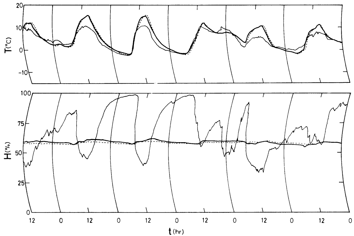
Fig. 5 住宅内気候の経時変化 (1973年12月18日～23日) 太線：合板内装，点線：珪酸カルシウム板内装，細線：百葉箱
