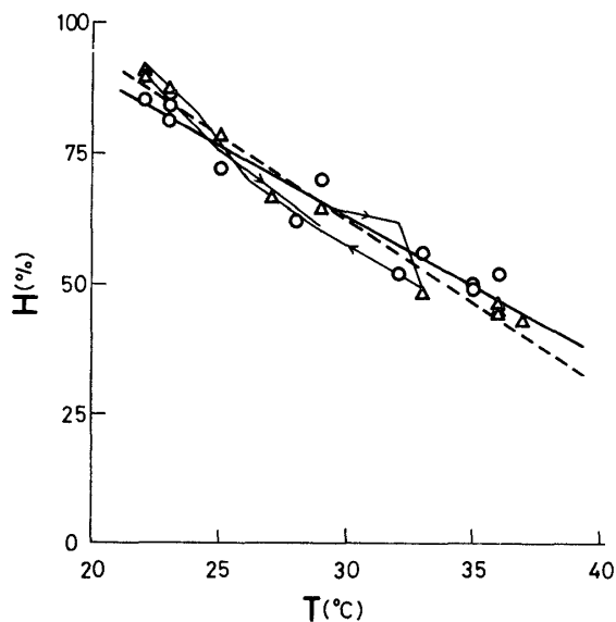
Fig. 28 湿度・温度の日変化(1974年8月15日) 白丸：合板内装，三角：メラミン美粧合板内装，細線：百葉箱，窓開放
