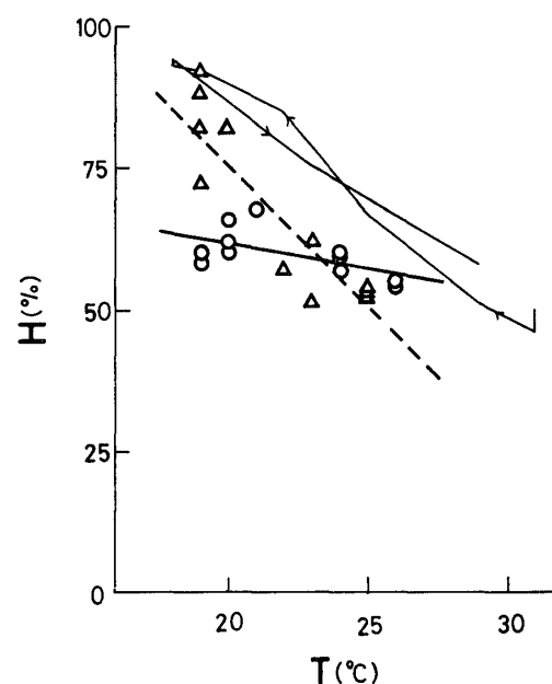
Fig. 25 湿度・温度の日変化(1974年8月8日) 白丸：合板内装，三角：メラミン美粧合板内装，細線：百葉箱，冷房時
