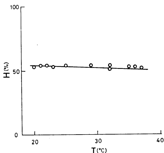
Fig. 33 湿度・温度の日変化（1974年6月12日） 白丸：インシュレーションボード内装（観測値），実線：計算値
