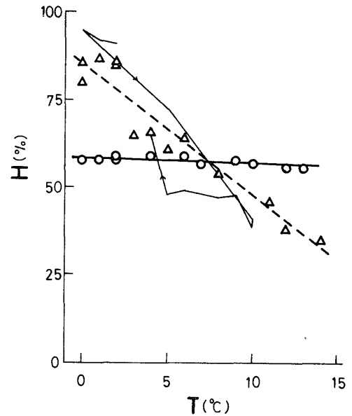
Fig. 21 湿度・温度の日変化(1974年1月23日) 白丸: 合板内装, 三角: ビニルシート 内装, 細線: 百葉箱
