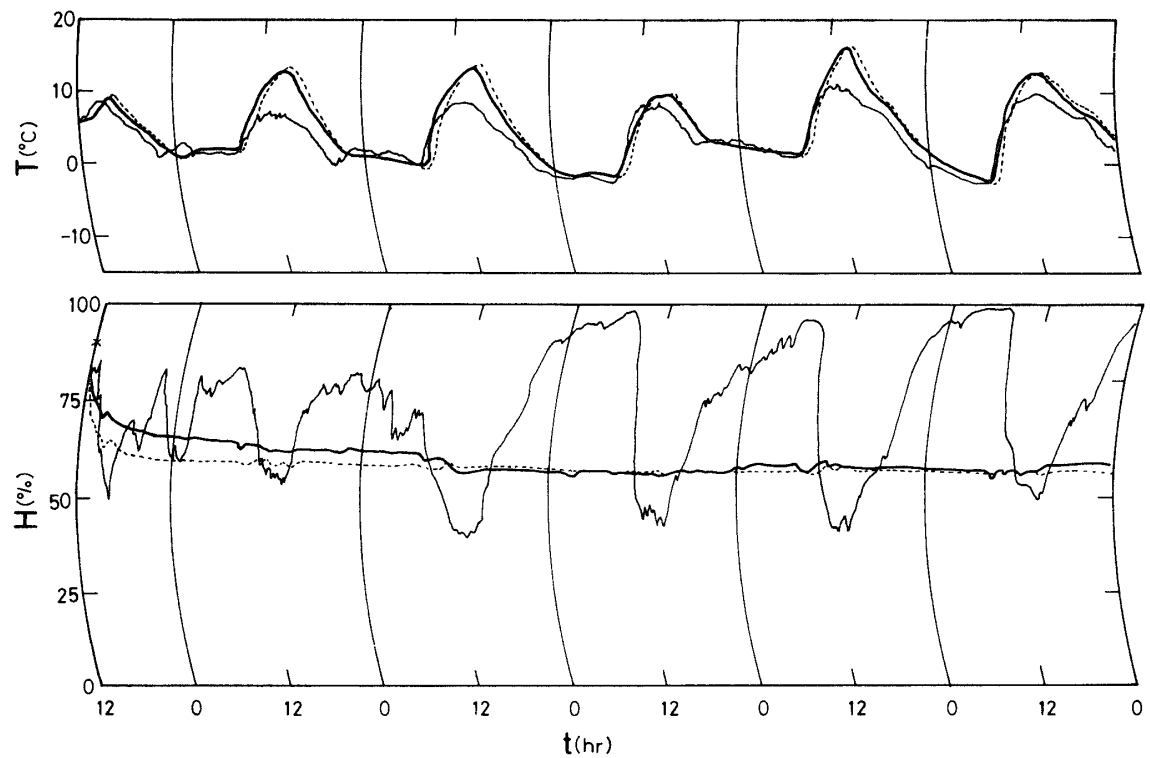
Fig. 6 住宅内気候の経時変化 (1973年12月28日～1974年1月2日) 太線：合板内装，点線：珪酸カルシウム板内装，細線：百葉箱
