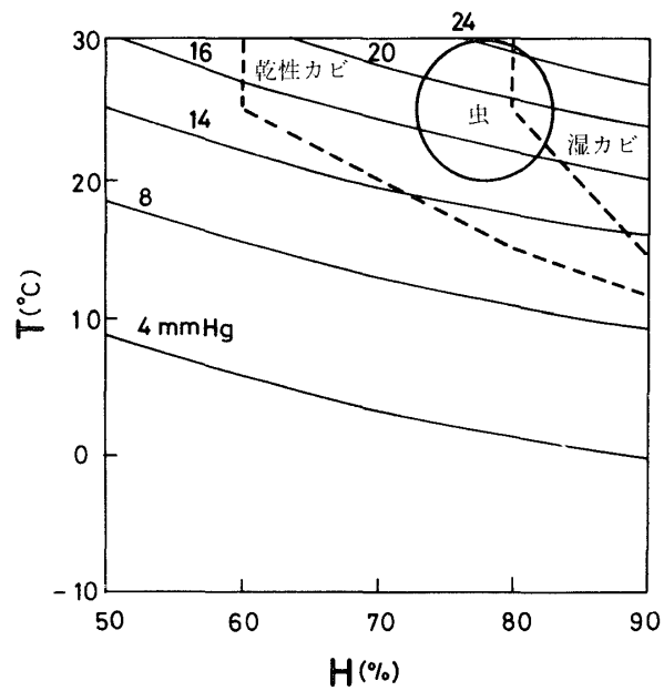
Fig. 2 等水蒸気張力線を有する気候図 1,4)
