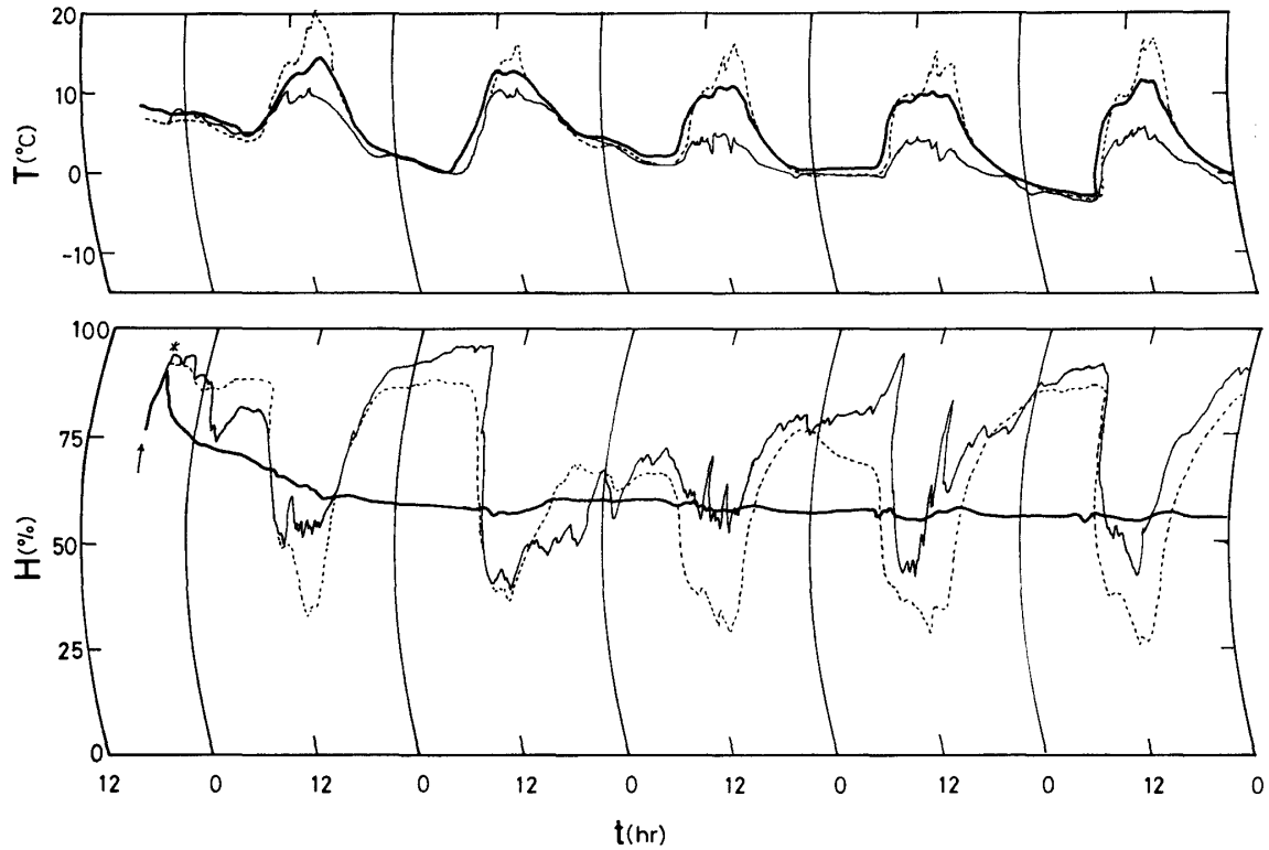
Fig. 7 住宅内気候の経時変化 (1974年1月21日～26日)
