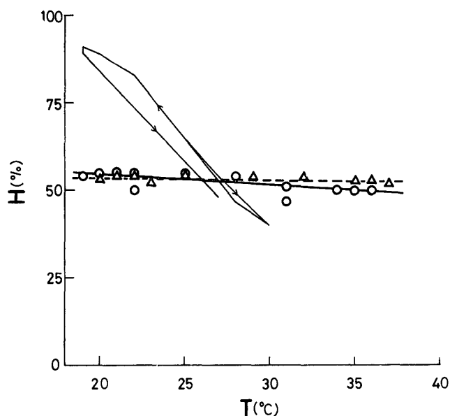
Fig. 23 湿度・温度の日変化(1974年6月12日) 白丸：合板内装，三角：インシュレーションボード内装，細線：百葉箱
