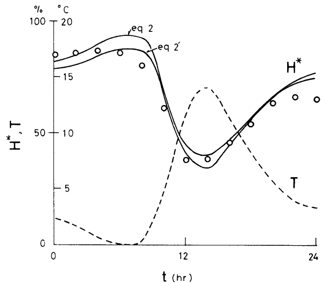
Fig. 31 ビニルシート内装住宅内湿度の日変化 (1974年1月23日) 白丸：観測値，実線：計算値（式②， ②'参照），点線：温度
