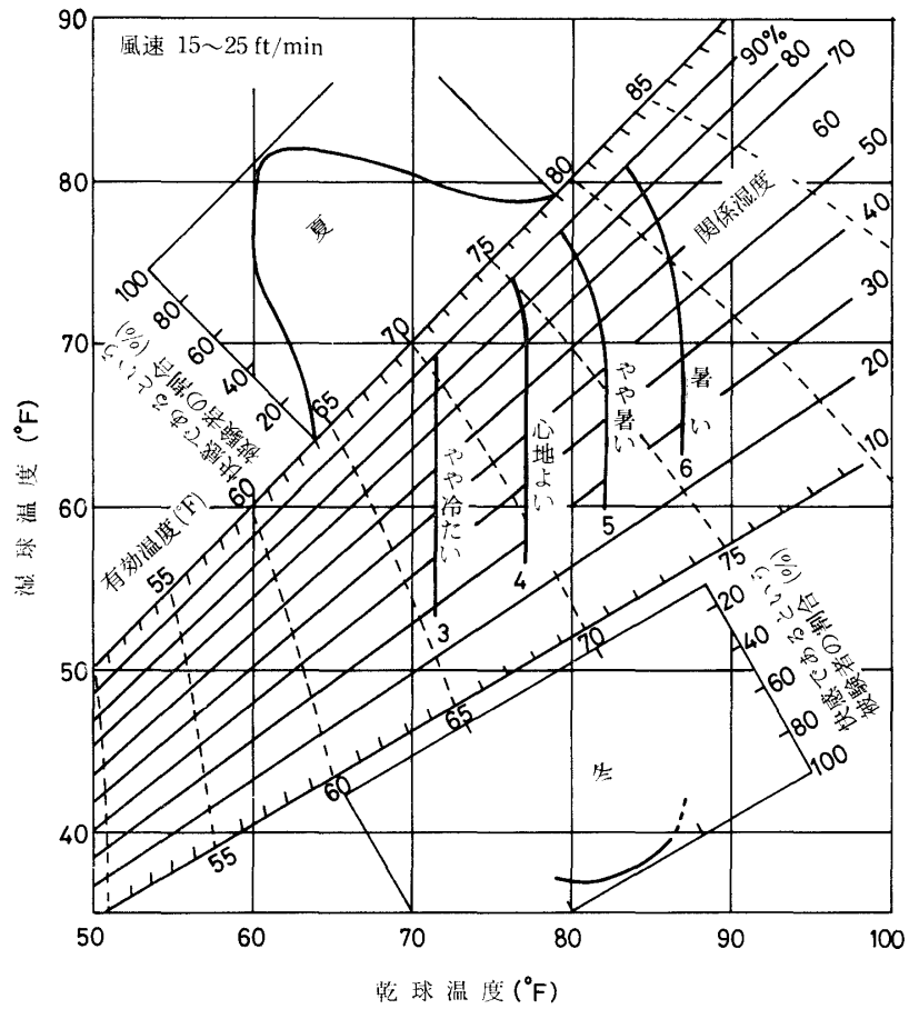
Fig. 1 修正 ASHRAE 快感図 1)
