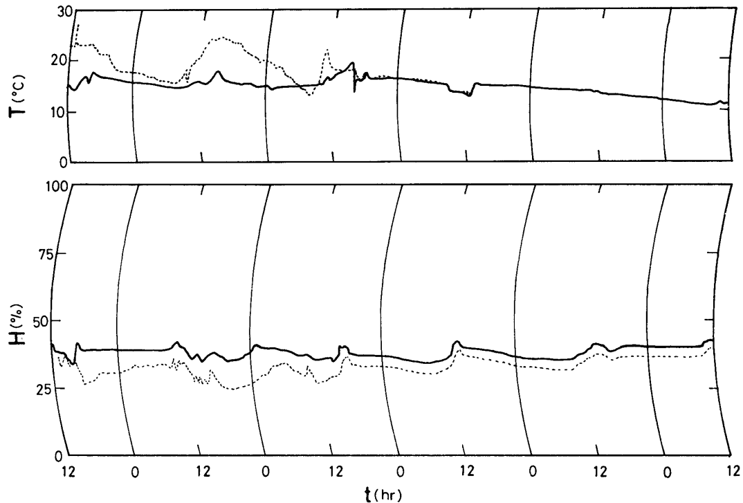
Fig. 19 研究所実験室（太線），研究室（点線）内気候の経時変化（1975年2月18日～23日）
