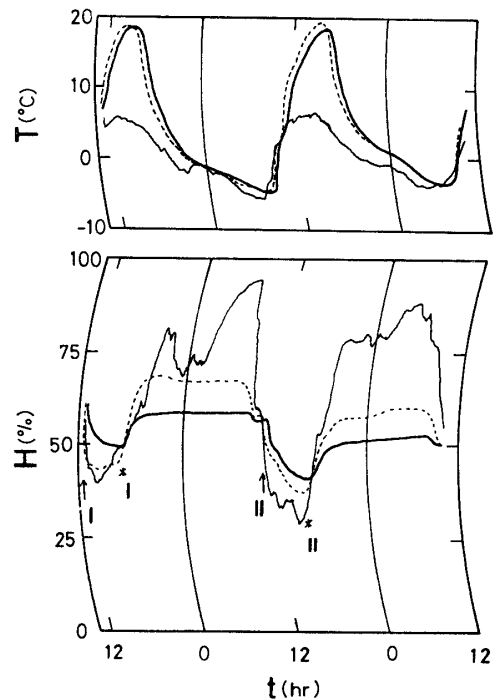
Fig. 18 住宅内気候の経時変化 (1975年12月15日~17日) 太線：合板内装，点線：床ビニールタイル，天井ロックウール，壁メラミン美粧合板内装，細線：百葉箱
