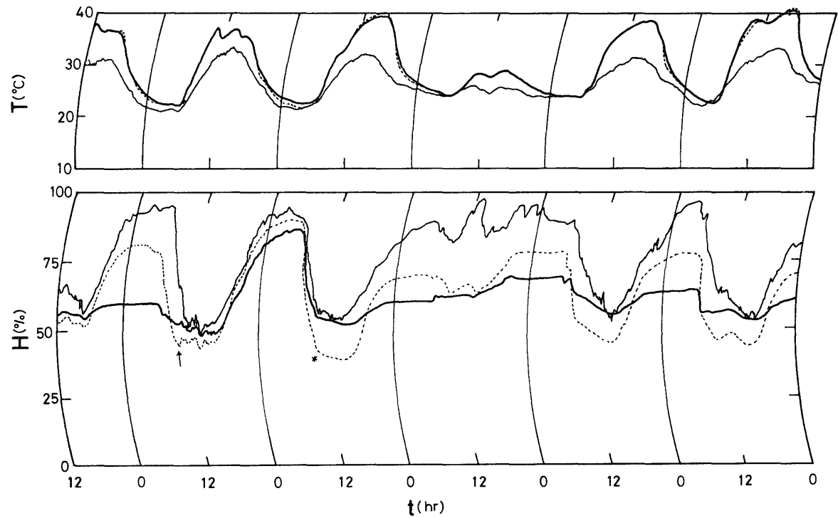
Fig. 14 住宅内気候の経時変化 (1974年8月14日～19日) 太線：合板内装，点線：メラミン美粧合板内装，細線：百葉箱
