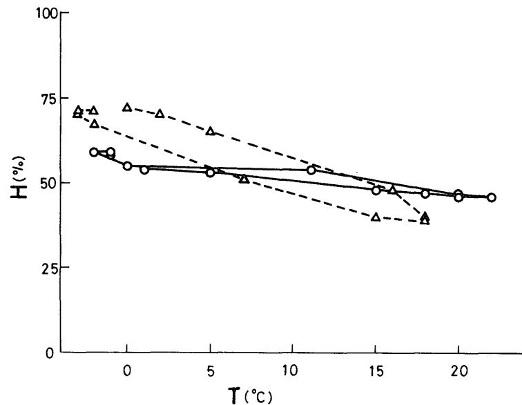
Fig. 27 湿度・温度の日変化 (1975年2月17日) 白丸：合板内装，三角：メラミン美粧合板内装，一時期暖房
