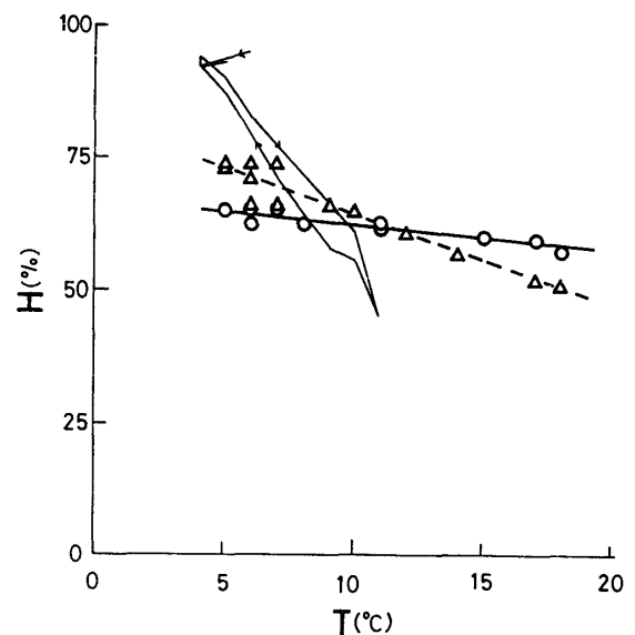
Fig. 29 湿度・温度の日変化(1975年11月30日) 白丸：合板内装，三角：天井ロックウール，床ビニルタイル，壁メラミン美粧合板内装，細線：百葉箱
