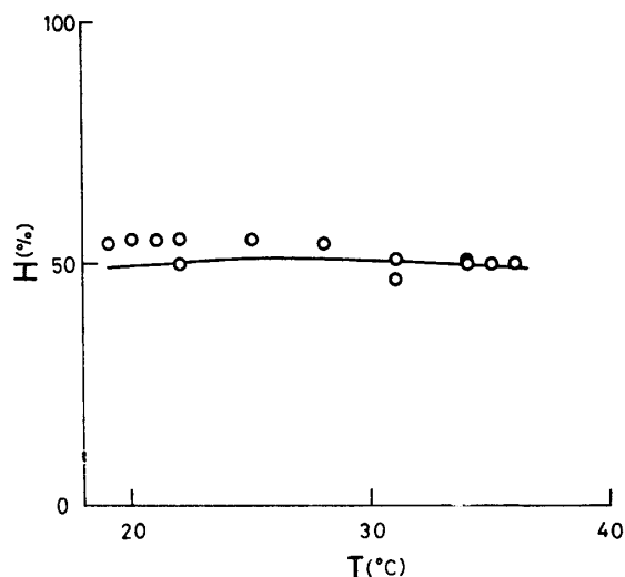
Fig. 32 湿度・温度の日変化（1974年6月12日） 白丸：合板内装（観測値），実線：計算値
