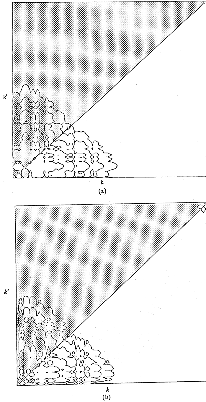
図 4: 乱流状態におけるエネルギー循環関数の等高線 ( L=48 )。
