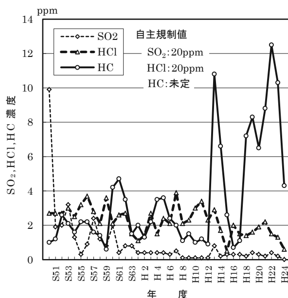
図6 KYS排出ガス平均濃度(排気筒出口) \text{SO}_2 , \text{HCl} , \text{HC}
