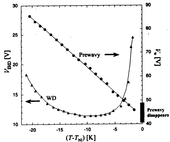
図7：prewavy パターンと EHD のしきい値電圧の温度依存性。
