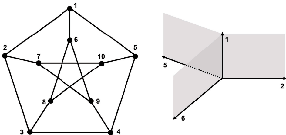
図2 (左): 系統樹空間 \mathcal{T}_4 = \mathcal{O}(\mathcal{E}^{(4)}, \Omega^{(4)}) に対する \Omega^{(4)} . 1, 2, ..., 10 とラベルが付けられているグラフの各頂点が \Omega の 1 点集合に対応し、線で繋がった 2 つの頂点の集合全体が \Omega に含まれる 2 点集合に対応する. (右): \mathcal{T}_4 の一部.
