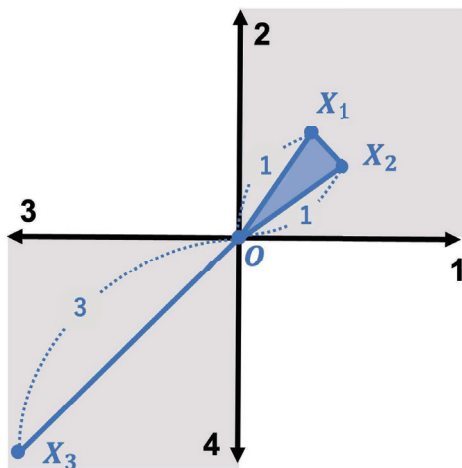
図3 最尤推定量が存在しない例.
