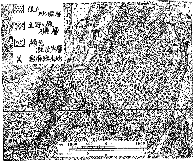
第一圖 小矢部川流域地質略圖
