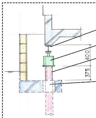
図-3.5 底盤を削孔しての押し込み
