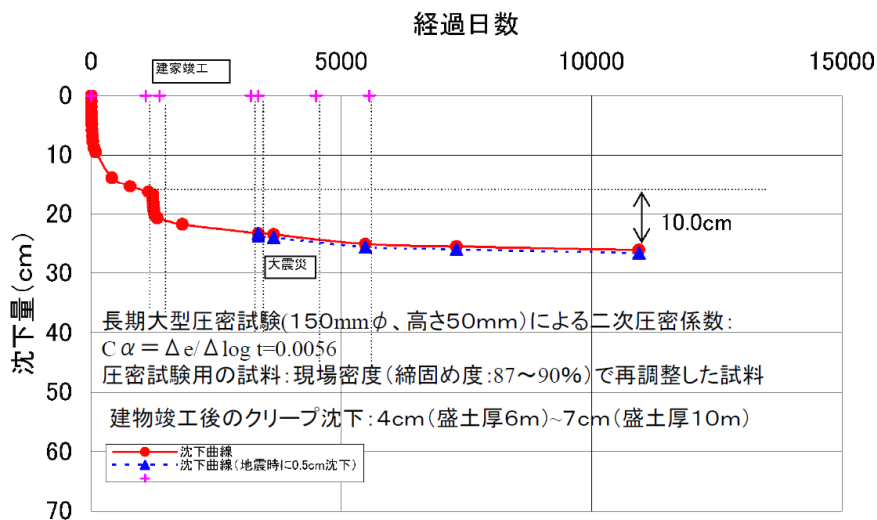
長期圧密試験結果に基づく沈下予測結果
