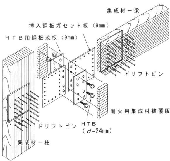
図 6：改良型鋼板挿入ドリフトピン接合
