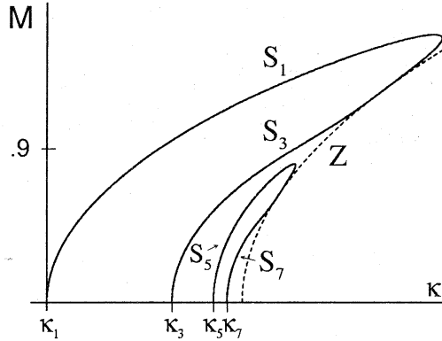
Fig. 2.3. The branches \mathcal{S}_1 , \mathcal{S}_3 , \mathcal{S}_5 and \mathcal{S}_7
