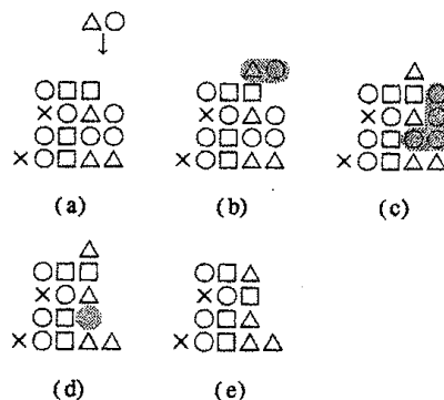
図 1 一般化ぷよぷよの操作の例
