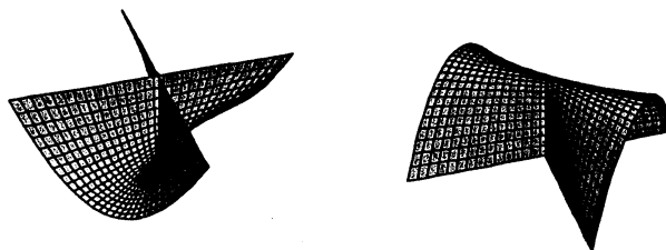
図 3: Whitney の傘
