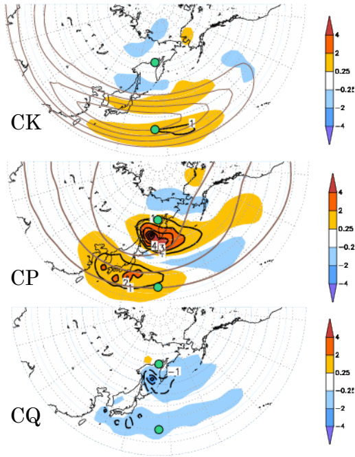
図 4. (上図)順圧エネルギー変換量 (CK), (中央図) 傾圧エネルギー変換量 (CP), (下図)非断熱加熱によるエネルギー生成量 (CQ)の鉛直積算図. 線、陰影ともに変換量 ( \text{W}/\text{m}^2 ). コンター間隔は 1 \text{ W}/\text{m}^2 . 上図 (中央図)の茶線は U250 (T500)の DJF 気候平均場. 緑点は WG81 による WP の定義位置.
