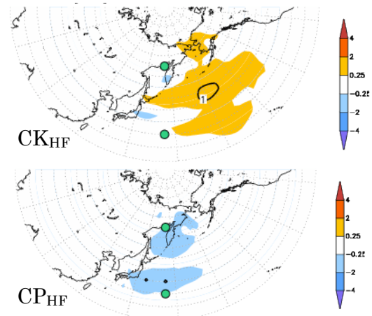
図 5. (上図)移動性擾乱に伴う順圧エネルギー変換量 ( \text{CK}_{\text{HF}} ), (下図)移動性擾乱に伴う傾圧エネルギー変換量 ( \text{CP}_{\text{HF}} )の鉛直積算図. 線、陰影ともに変換量 ( \text{W}/\text{m}^2 ). 上図. 緑点は WG81 による WP の定義位置.
