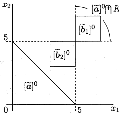
図 1: 0-レベル集合
