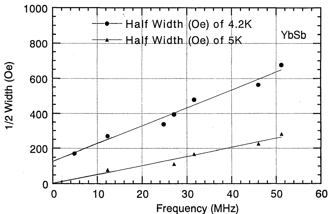
図5 転移温度以上と転移温度以下でのスピンエコースペクトルの半値幅の周波数依存性
