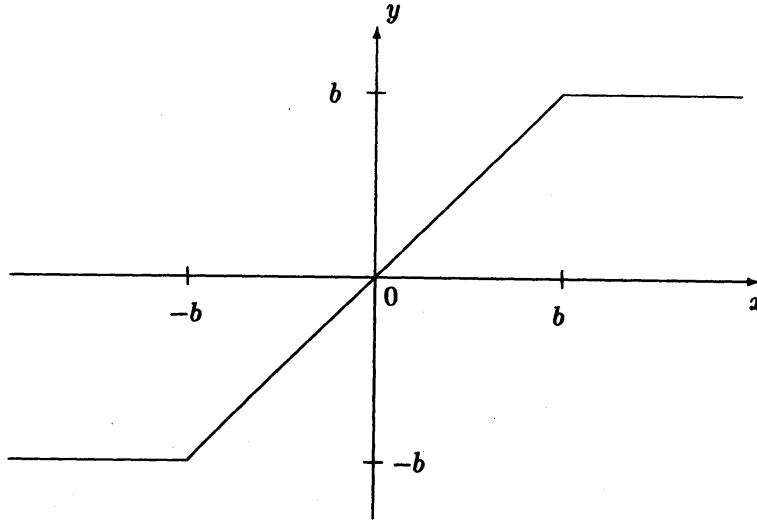
図1 関数 \psi(x)
