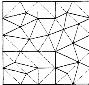
図 2: メッシュ例 ( N_\Omega = 5 )
