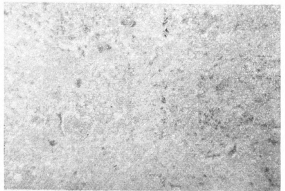
図4 組織像
