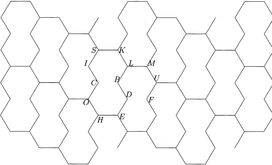
図 18: パターン IV_3 の部分パターン X_1
