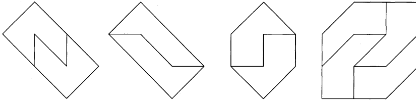
図 61: 半方 IV 図の図形 11, 14, 7, 8 のパターンの基本図形
