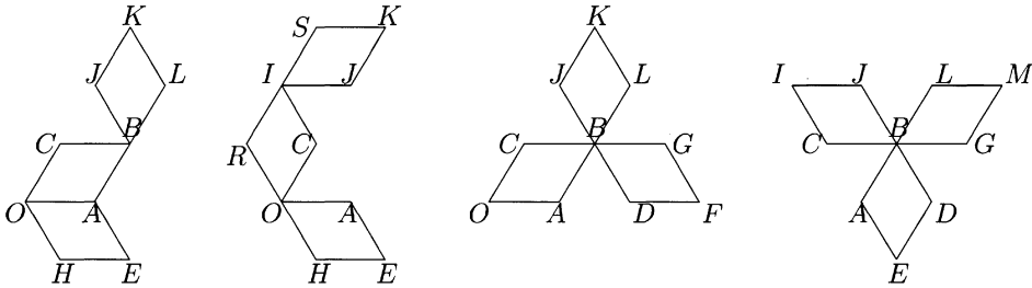
図 22: パターン IV_3 の平行移動群の基本図形
