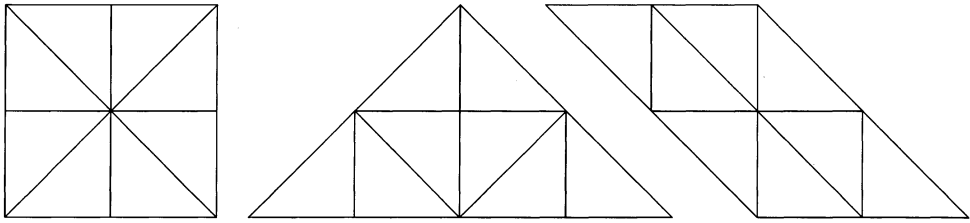
図 55: 倍の大きさには 4 倍の個数の定規が要る (平方Ⅱ×2)
