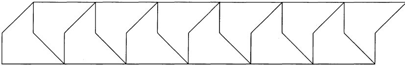
図 63: 半方 IV 図の図形 5 のパターン 1
