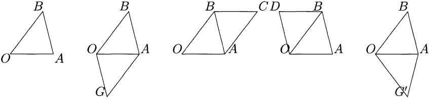
図 43: 一般の三角形のかっつき方
