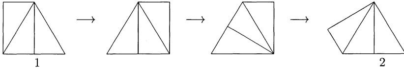
図 71: 半正 III 図の図形 1 と図形 2 は組み合わせ図形としては同じ
