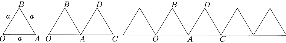
図 8: 正三角形を左右へ
