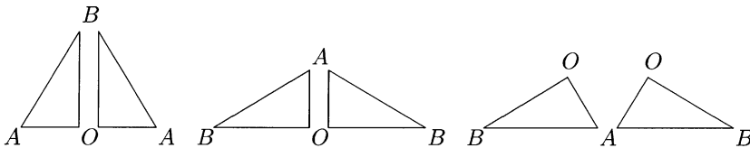
図 67: 半正三角形の6つの置き方 (半三 I)
