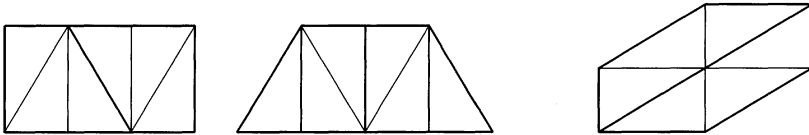
図 72: 半正 III 図の図形 1 のパターンの 2 次の部分パターンの基本図形
