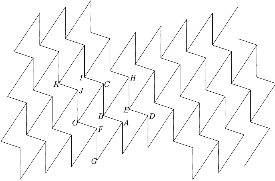
図 41: 六角形のパターン VI_6
