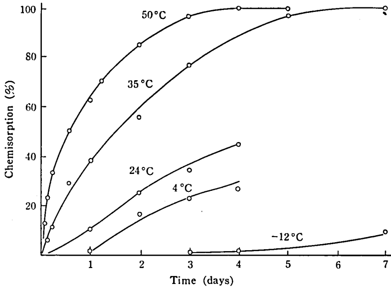
図9. \text{PH}_3 の化学的吸着におよぼすくん蒸温度と時間の影響 70)
