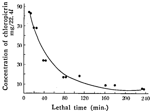
図 4. CP 濃度とマウス致死時間の関係 30)
