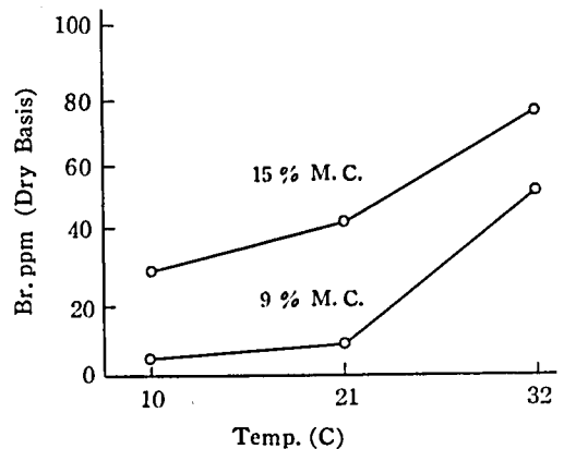
図 7. 水分含量と温度の残留量におよぼす影響 57)
