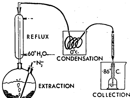
図 10. Acid Reflux 法で用いた抽出装置 90)
