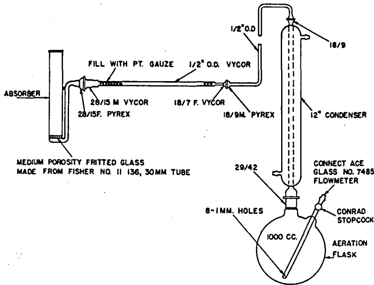
図 11. 残留 C.P. 抽出装置 65)
