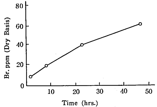
図 6. くん蒸時間の残留量におよぼす影響 57)
