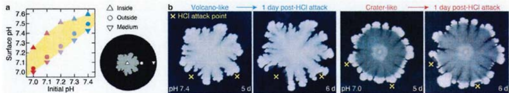
図 1: 環境 pH 変化とコロニーの防御性能。a, 接種 5 日後における表面 pH の分布。コロニー内部方向に向かって pH は上昇している。b, 短期的 pH 変動に対するコロニー形態の防御性。接種 5 日後のコロニーに対して、コロニー境界のすぐ外側の x 印の点に 10 \mu l の 2.4 g l -1 塩酸を滴下した。塩酸はすぐに培地内を拡散するが、少量のために長期的な pH 変化は 0.04 未満で無視できる程度である。すなわち、短期的な環境変動の影響を調べた。主にクレーター型形態によく見られる壁構造の付近では被害 (成長先端領域の細胞のコロニー内側への回避) が小さい。
