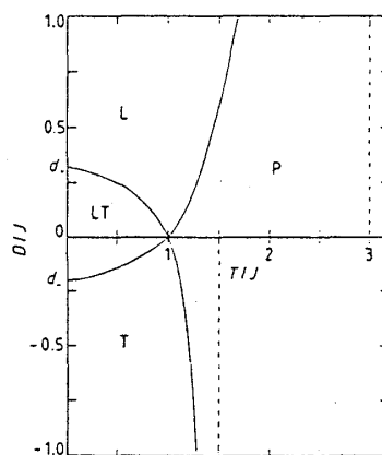
Fig. 4 D/J の磁気状態図
