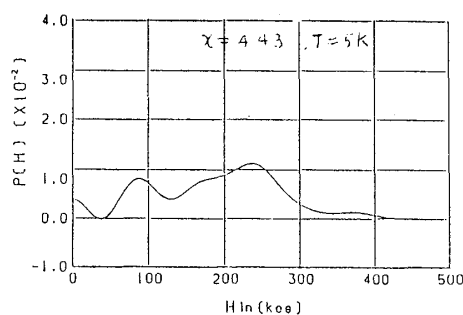
Fig. 14 x=4.43 の5Kにおける内部磁場分布
