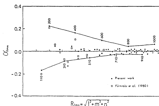
Fig. 6 x=0.20 の \alpha(R_{lmn})
