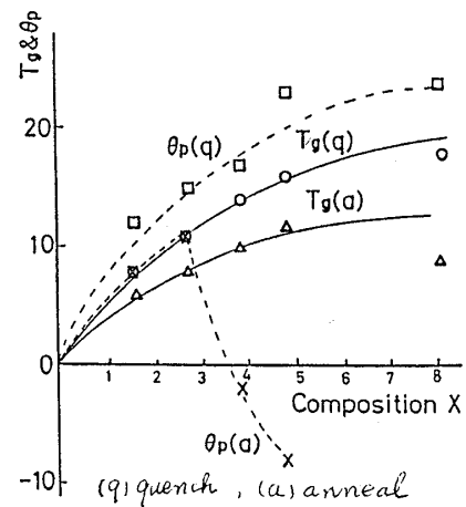
Fig. 11 \text{Cu}_{100-x}\text{Fe}_x の \theta_p(x) と T_g(x)
