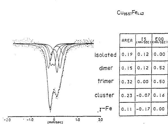
Fig. 12 x=4.43 の常磁性スペクトル
