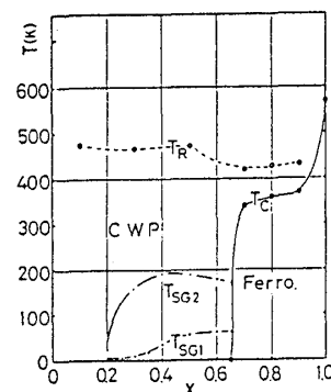
Fig. 3 Ni_{1-x}Mn_xSb の磁気状態図
