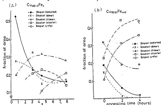
Fig. 13 Fe集合体の組成および熱処理依存性
