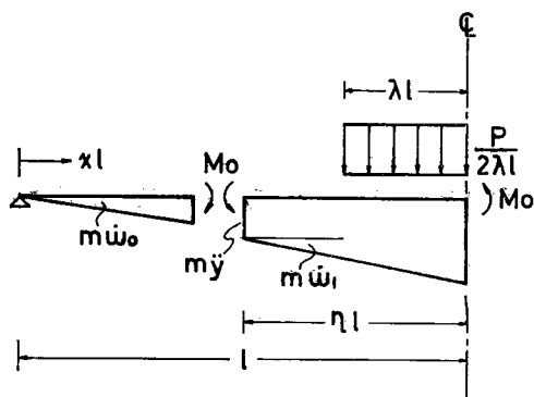
Fig. 6 Type A' Motion
