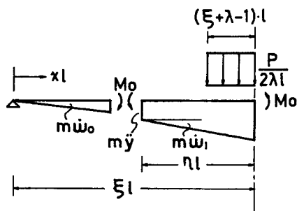
Fig. 7 Type B' Motion
