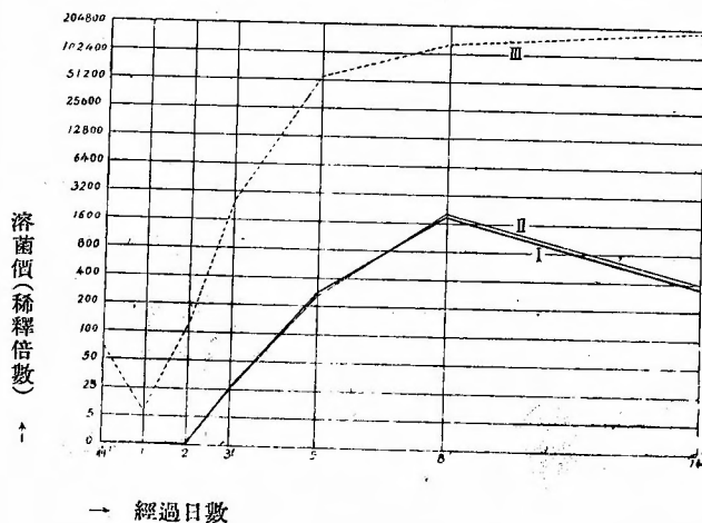
第1圖 溶菌價ノ時間的推移 (第1表參照)
