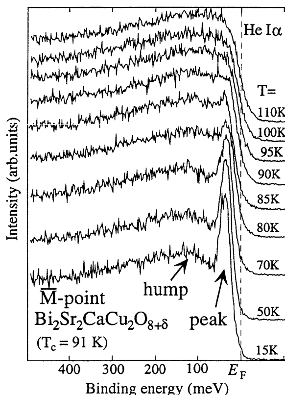
図2 最適ドーピングBi2212( T_c=91\text{K} )のM点における光電子スペクトルの温度変化
