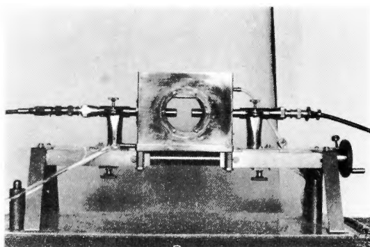
図11 測定容器
