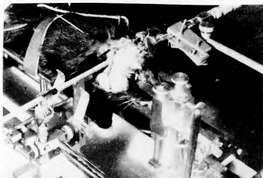
図18 透過法による猫腎の超音波減衰度測定
