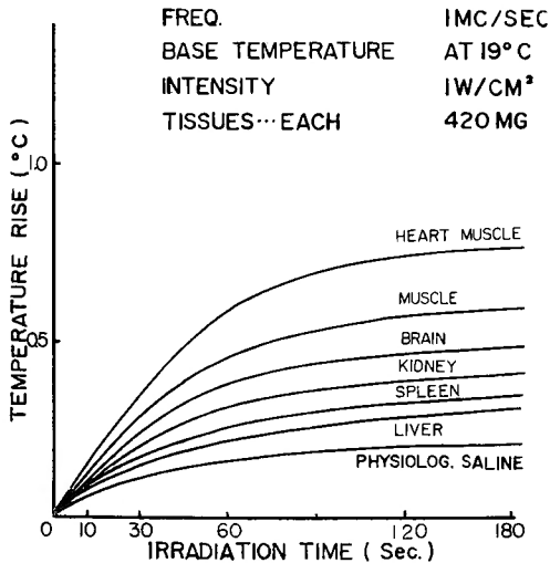
図25 マウス各臓器の温度上昇 (ホモゲナイズした組織)
