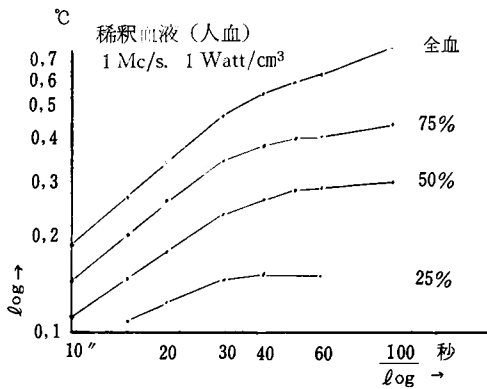
図24 超音波照射時間と温度上昇の関係
