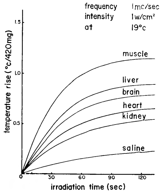
図26 マウス各臓器の温度上昇
