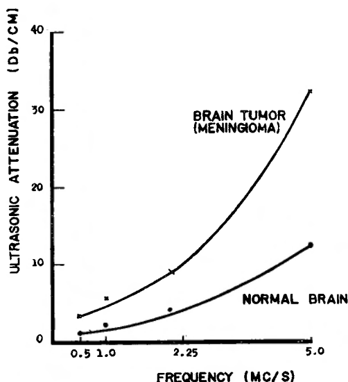
図28 透過法により測定した正常脳組織と脳腫瘍組織の超音波減衰度
