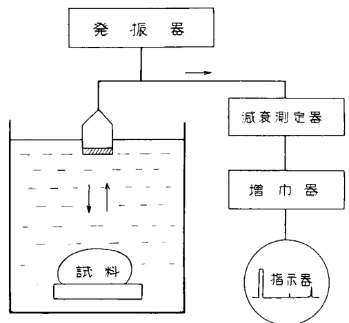
図1. 超音波反射法による減衰測定法（水浸法）
