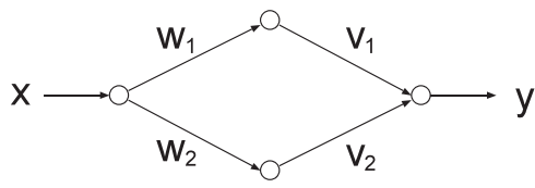
図 1: 中間層に 2 つのニューロンを持つ 3 層パーセプトロン: ノードは活性化関数 \tanh(\cdot) . エッジはパラメーター \theta = (w_1, w_2, v_1, v_2) による線形重ね合わせを表す. 出力 y は入力 x とパラメーター \theta の関数 f(x; \theta) で与えられる.
