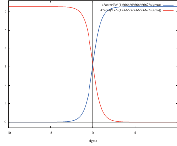
図 1 左が反キンク, 右がキンク, v = 0.5
