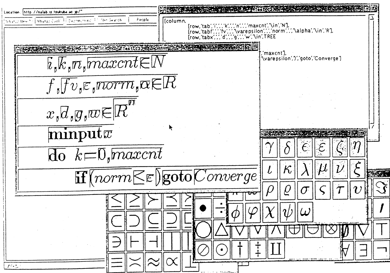
図2 nMath-p 画面例
