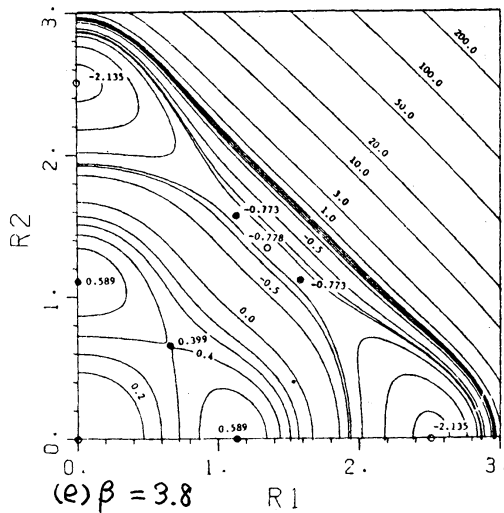
図9 平均ポテンシャルの等高線図 \circ : 極小点 (安定平衡点) \bullet : 鞍点, 極大点 (不安定平衡点)
