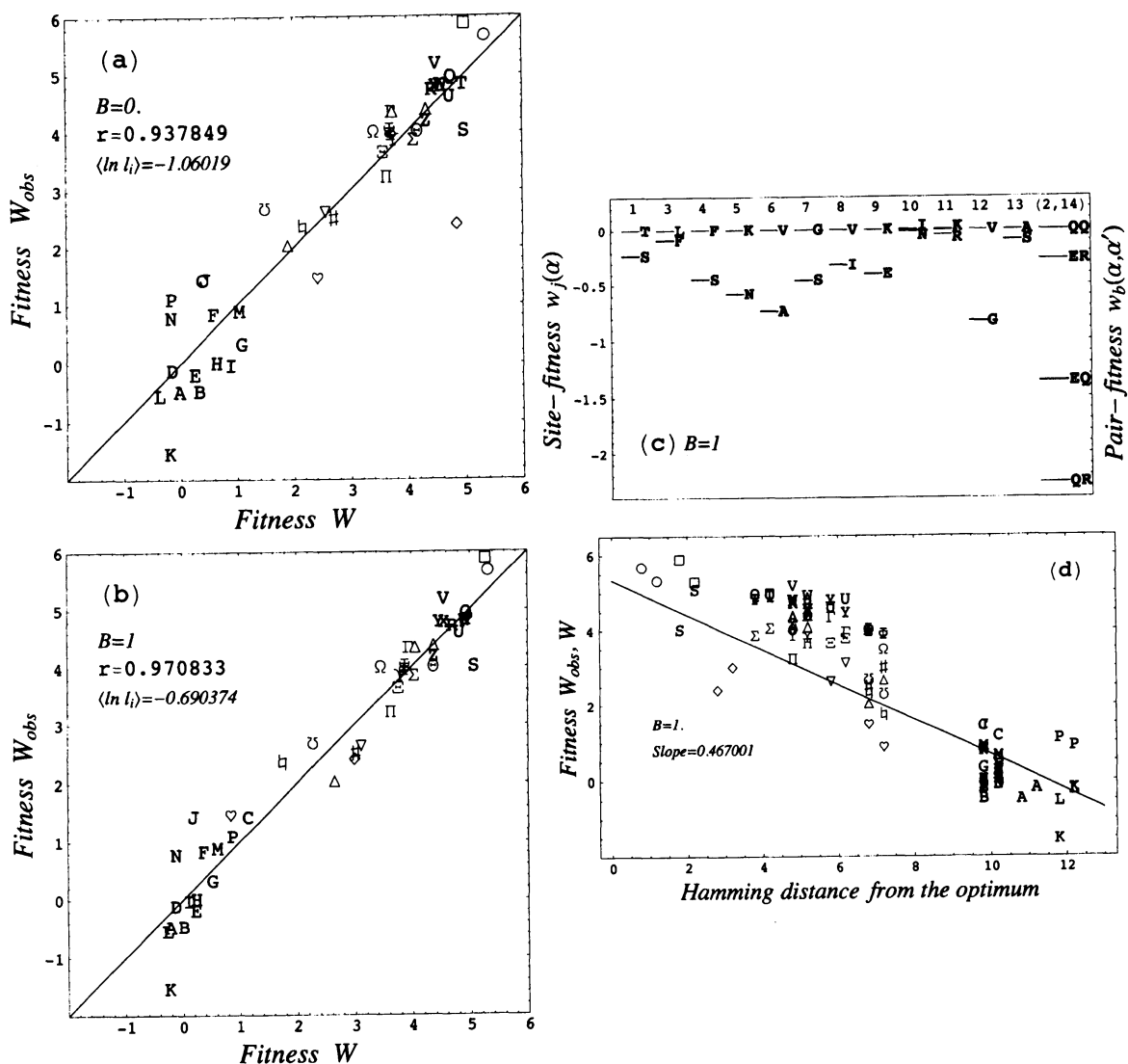
図 3: プロリルエンドペプチダーゼの耐熱性の地形の解析結果. (a,b) 縦軸は適応度の実測値 W_{\text{obs}} 、横軸はパラメータ適合で得た適応度の値 W . (a) は式 (1) の適応度関数を用いた場合で、(b) は式 (2) の適応度関数を用いた場合. 各シンボルは 45 種類の各クローンに対応する. r は相関係数. (c) 式 (2) の適応度関数を用いた場合に決定されたパラメータの値. 左から 1~13 のレーンは部位の寄与 w_j(x_j) を表し、一番右側のレーンは残基ペアの寄与 w_b(x_k, x_l) を表す. 図の上部に示した数字は解析のための部位の通し番号である. アルファベットは一文字表記のアミノ酸を表す. 一番右のレーン (2,14) においては、"EQ" は、部位 2 が E (グルタミン酸) で部位 14 が Q (グルタミン) の意味であり、このペアは野生型残基ペアである. これら 2 つのいずれかが変異型残基 ("ER"、"QQ") になると適応度が大きく増大するが、両方とも変異型残基 ("QR") になると適応度は激減する. (d) 配列空間を 1 次元軸 (最適配列からのハミング距離) へ投影することによる適応度地形の表現. 各ハミング距離の位置において、左列の文字は実測値 W_{\text{obs}} を、右列の文字はパラメータ適合で得た適応度の値 W を表す. 斜線は地形の平均勾配を表す. (文献 [6] より転載)
