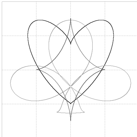
図 2: plotover
