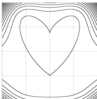
☒ 9: conplotQ(H)
