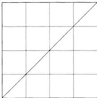
図 4: ifplotQ
