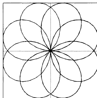
図 7: polarplot
