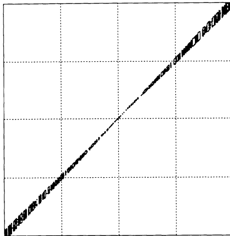
図 1: ifplot による (x-y)^{10} の図
