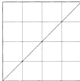
図 5: ifplotB
