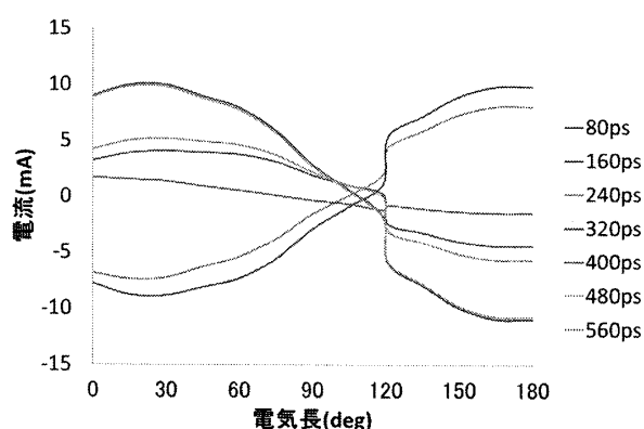
図4 基本波の電流定在波
