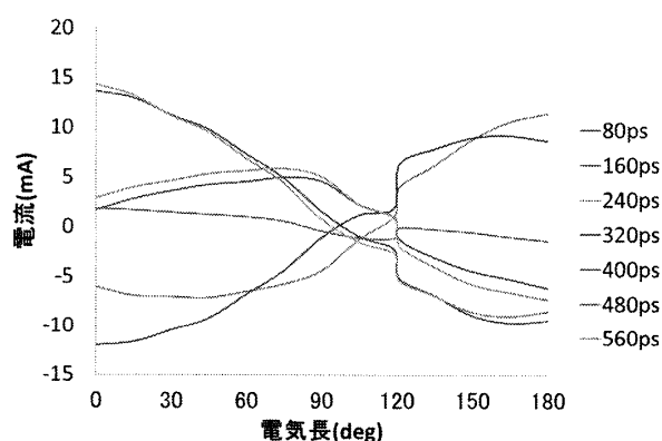
図3 電流定在波
