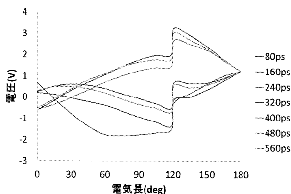
図2 電圧定在波
