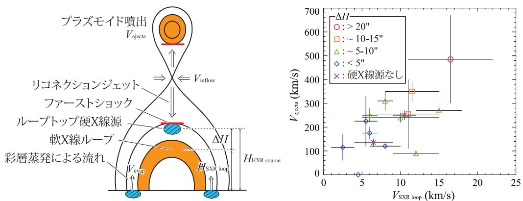
左図: フレアのリコネクションモデル。右図: 軟 X 線ループの上昇速度 ( V_{\text{SXR loop}} ) とプラズモイド噴出の速度 ( V_{\text{ejecta}} )、ループ上空の硬 X 線源の高さ ( \Delta H ) の関係。
