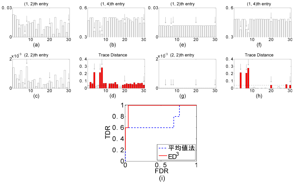
図2 シミュレーションデータの結果一例：(a)–(d) 観測行列の (1, 2), (1, 4) 及び (2, 2) 要素と平均値法により計算されたトレース距離（図中の矢印は異常行列），(e)–(h) ED^3 により計算された行列の (1, 2), (1, 4) 及び (2, 2) 要素とトレース距離（図中の矢印は異常行列），(i) 平均値法と ED^3 の ROC 曲線
