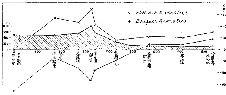
興安嶺横斷重力偏倚分布圖
