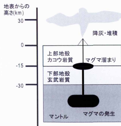
図1 火山の概念図
