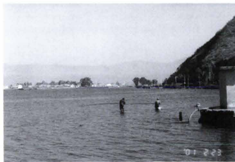
写真2 星雲湖
