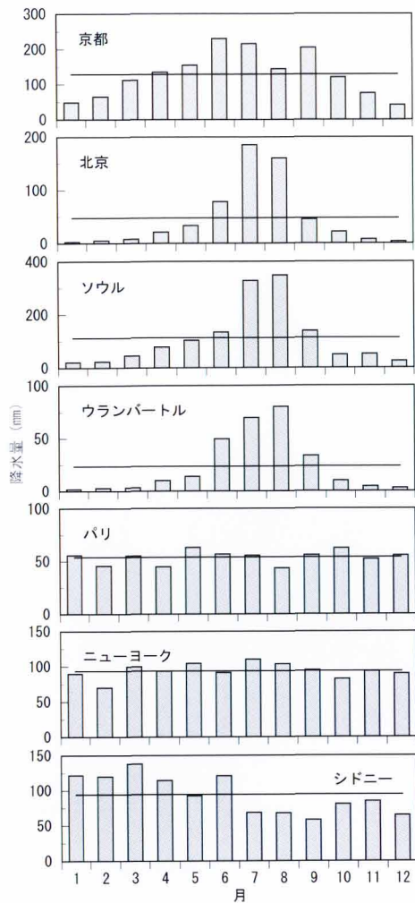
図2 月別降水量の季節変化 理科年表(2008)。図中の直線は年間の平均値。
