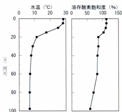
図1 停滞期における琵琶湖での水温と溶存酸素飽和度の鉛直分布 今津沖（水深98.7m）。2006年8月21日。 滋賀県琵琶湖環境科学研究センターの観測値をもとに著者作図。
