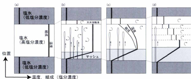
図2 実験の結果。(a)～(d)まで時間順に並んでいる。図中の太い実線および点線はそれぞれ鉛直方向の温度、組成（塩分濃度）を示す。(a)初期状態。(b)実験開始直後。活発な対流により均質な二層。(c)下の液層では、次第に上ほど温度が低く、塩分濃度が低い温度組成勾配ができる。(d)下の液層が多層に分かれて対流する。
