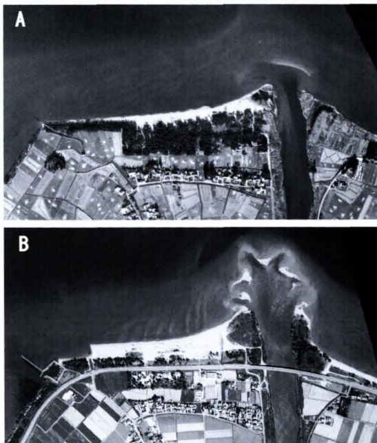
図10 航空写真における佐波江浜の地形の変化。
