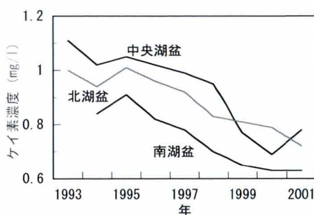
図8 バイカル湖での平均ケイ素濃度の減少 Shimaraev and Domysheva (2004)。
