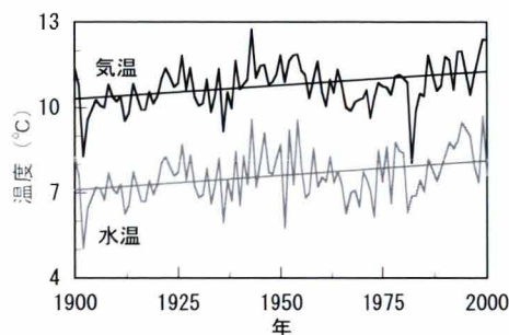
図7 バイカル湖南湖盆での気温と表面水温の推移 図中の直線は最小二乗法による近似直線。 Shimaraev and Domysheva (2004)。
