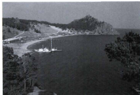
写真5 バイカル湖
