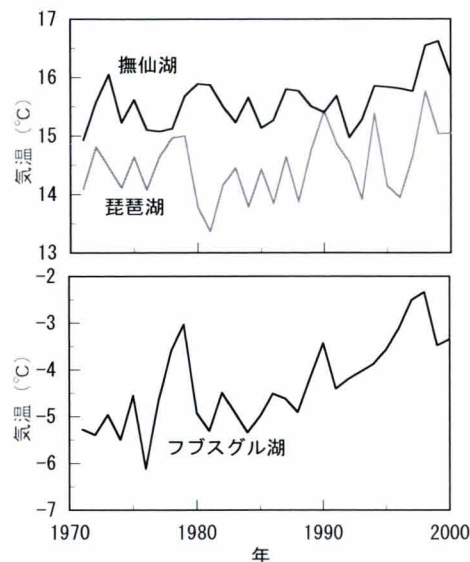
図6 湖での気温の変化 坂本充、熊谷道夫 (2006)。
