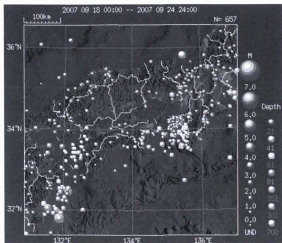
大阪管区気象台による地震分布
