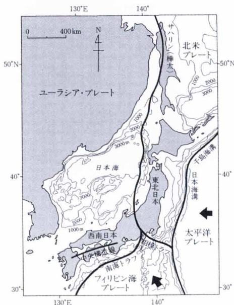
プレートの図
