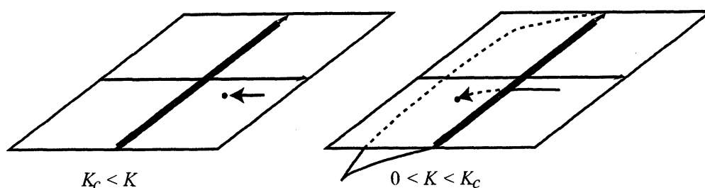
Fig. 2 パラメータ K を減らしていったときの固有値の動き。 K > K_c のときは普通の意味での固有値として存在しているが、 0 < K < K_c のときは複素平面とは異なる Riemann 面のシート上にあり、一般化固有値になる。
