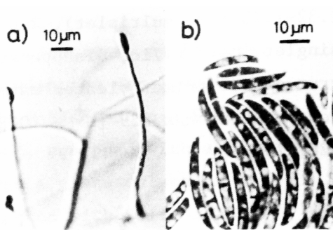
Fig. 2. a) Microconidia of F. solani TG-2. b) Macroconidia of F. solani TG-2.
