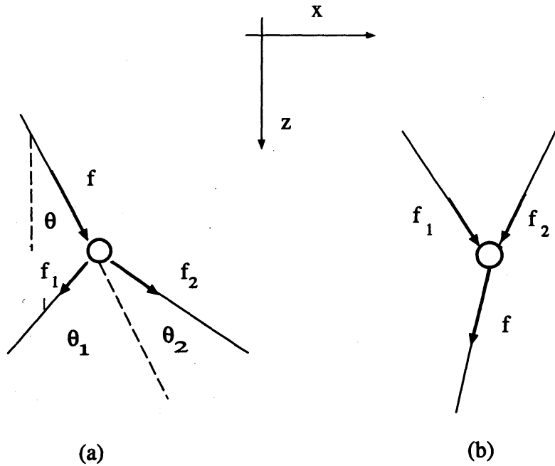
図 1: 不純物による force chain の散乱のモデル. (a) 分裂プロセスと (b) 合流プロセス.
