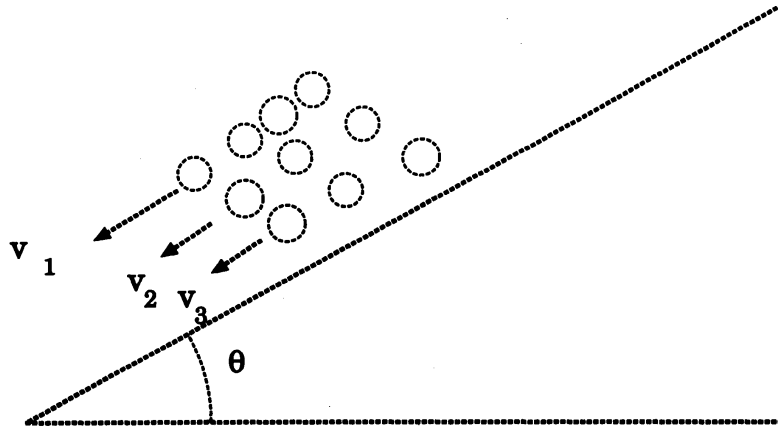
図 3: 斜面上の流れの概念図. 斜面上に鉛直方向にしか位置依存性がないときは 1 層目と 2 層目の相対速度は v_1 - v_2 となっていることに注意. 従って本文中にあるような展開が使える.
