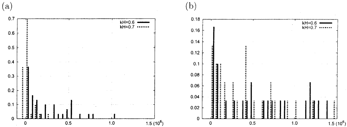
図 4: ヌクレオチドが解離してからミオシンが near-rigor 構造に緩和するまでの時間 (ステップ数) t_{\text{diff}} の分布 (サンプル数: 30). kH はヌクレオチドとタンパク質の相互作用の強さを決めるパラメータ. (a) 二面角ポテンシャルがある場合. 結合が強い場合には, 解離と緩和が同時に起こる傾向が強くなる. kH=0.7 のとき, t_{\text{diff}} < 0 のデータが多数あるが, ヌクレオチドが結合したまま緩和したわけではなく, 実際に時系列を見てみると解離と緩和が同時に起こっている. (b) 二面角ポテンシャルがない場合. kH に依らず, 構造緩和は解離とは同期していない. (但し, ヌクレオチドが解離しないと緩和しないという点では同じ.)
