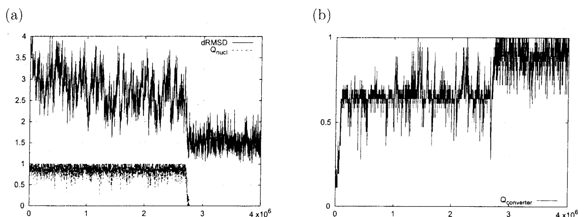
図 3: あるサンプルについての時系列データ. (a) 最終構造からの dRMSD と、タンパク質とヌクレオチドとの結合を表す指標 Q_{\text{nucl}} ( Q_{\text{nucl}} = 0 で解離). (b) コンバータ部に着目した指標. Q_{\text{converter}} = 1 のとき、「コンバータ部の他の部位に対する相対的な位置」が最終構造と同じになる.
