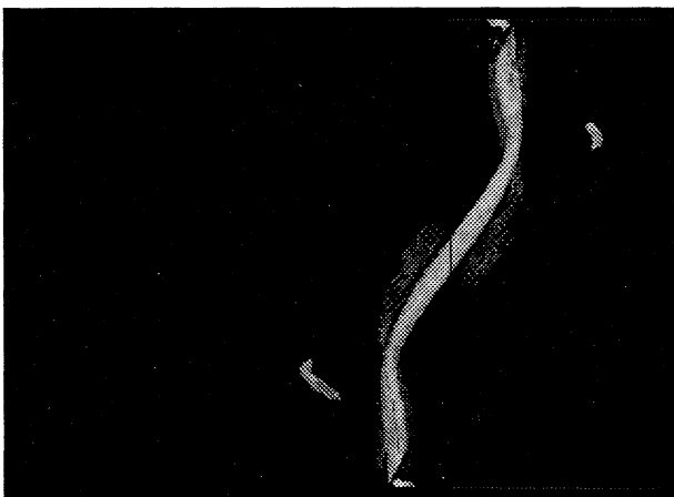
図4: エンストロフィー |\omega(x)|^2 (白) とエネルギー散逸 S^2 = S_{ij}S_{ij} (灰) の等値面 (上) t = 1.2 , (中) t = 2.0 , (下) t = 2.8 . 図5: |\omega^+(x)|^2 (白) と |\omega^-(x)|^2 (灰) の等値面 (上) t = 1.2 , (中) t = 2.0 , (下) t = 2.8 .
