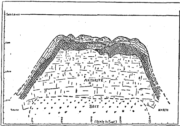
第三圖 アナイルナ州硫磺鹽丘斷面圖
