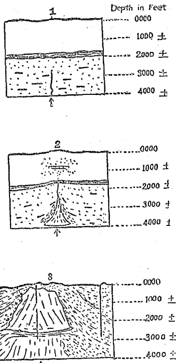
圖四第 第四圖 沈澱説鹽丘成因說明圖
